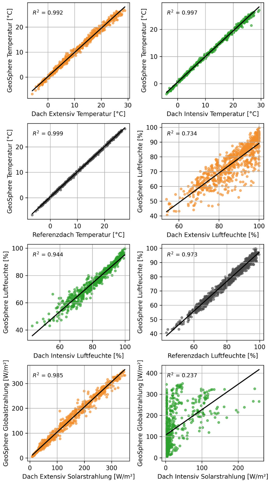
Abbildung 33: Regressionen der Tagesmittelwerte von Lufttemperatur, relativer Luftfeuchtigkeit und solarer Einstrahlung zwischen den untersuchten Wetterstationen HTL St. Pölten Extensivdach (EX), Intensivdach (INT), Referenzdach (REF) und der Geosphere Landhaus St. Pölten (GS) (© IBLB).
