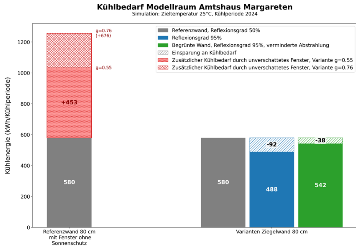
Abbildung 38: Kühlbedarf und Einsparung, Simulationsergebnisse: Vergleich mit Fenster ohne Sonnenschutz; Fassadenbegrünung troggebonden, W. sinensis , Amtshaus Margareten [FB1-tW] (© IBO).
