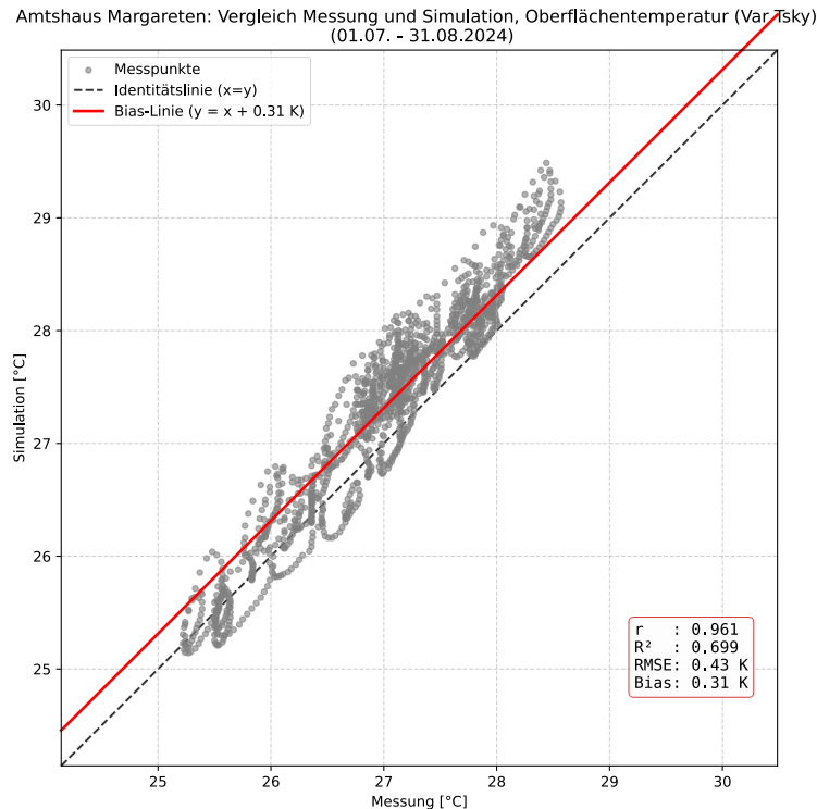
Abbildung 36: Scatterplot Juli-August 2024, Oberflächentemperaturen; Fassadenbegrünung troggebonden, W. sinensis , Amtshaus Margareten [FB1-tW] (© IBO).
