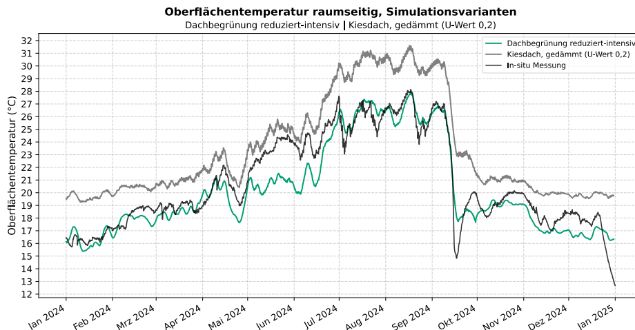
Abbildung 43: Temperaturverläufe der Simulationsvarianten zu in-situ Messung; reduziert-intensive Dachbegrünung, HTL St. Pölten [DB2-ri] (© IBO).
