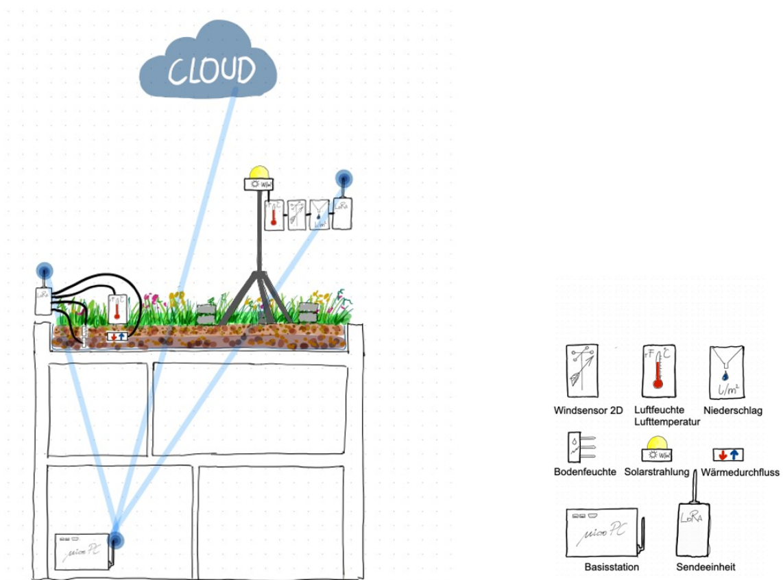
Abbildung 3: Messkonzept Fassadenbegrünungen, Beispiel extensives Gründach (© IBLB).
