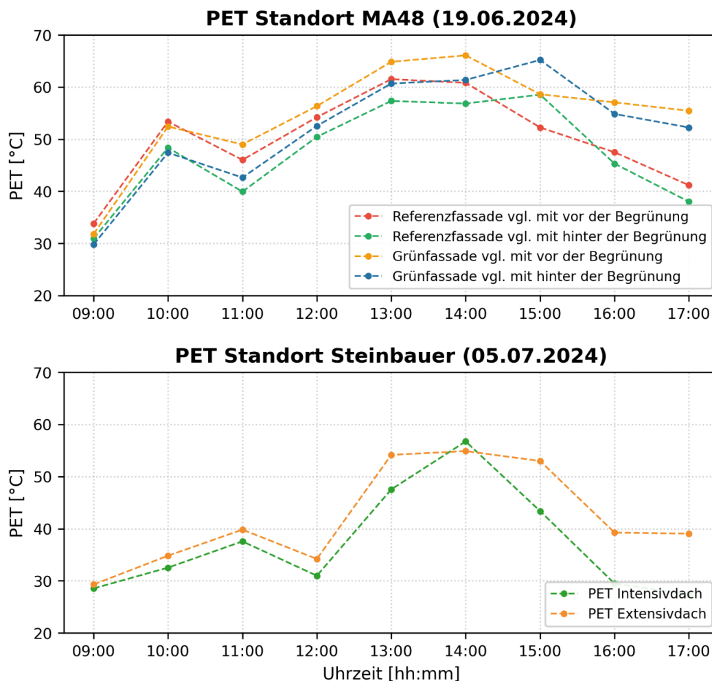
Abbildung 66: Tagesgänge der physiologisch äquivalenten Temperatur (PET) an zwei Standorten. Oben: MA48 [FB4-w] am 19.06.2024 mit Referenzfassade und Grünfassade, jeweils „vor“ und „hinter“ der Begrünung; Unten: Steinbauer am 05.07.2024 mit Intensiv- und Extensivdach [DB1-e, DB1-i] (© IBO).
