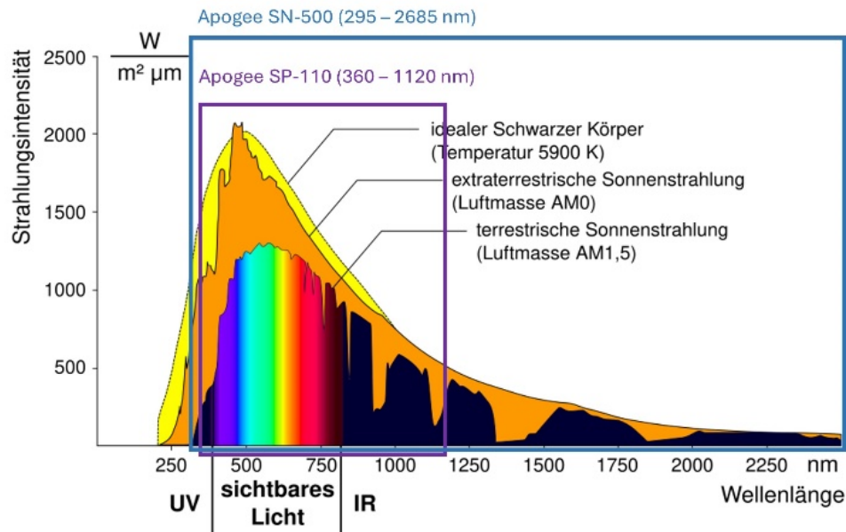
Abbildung 11: Strahlungsintensität der Sonnenstrahlung mit Strahlungssensor Spektrum (Bildquelle: wikicommons, verändert).
