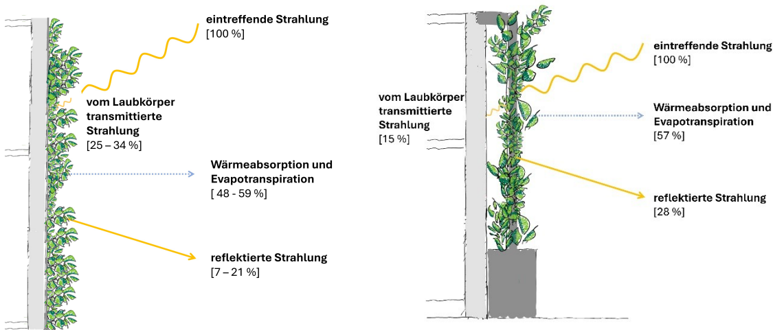
Abbildung 71: kurzwellige Strahlungsbilanz als Mittelwerte der in 2024 untersuchten boden- und troggebundenen Begrünungsobjekte (© IBLB).
