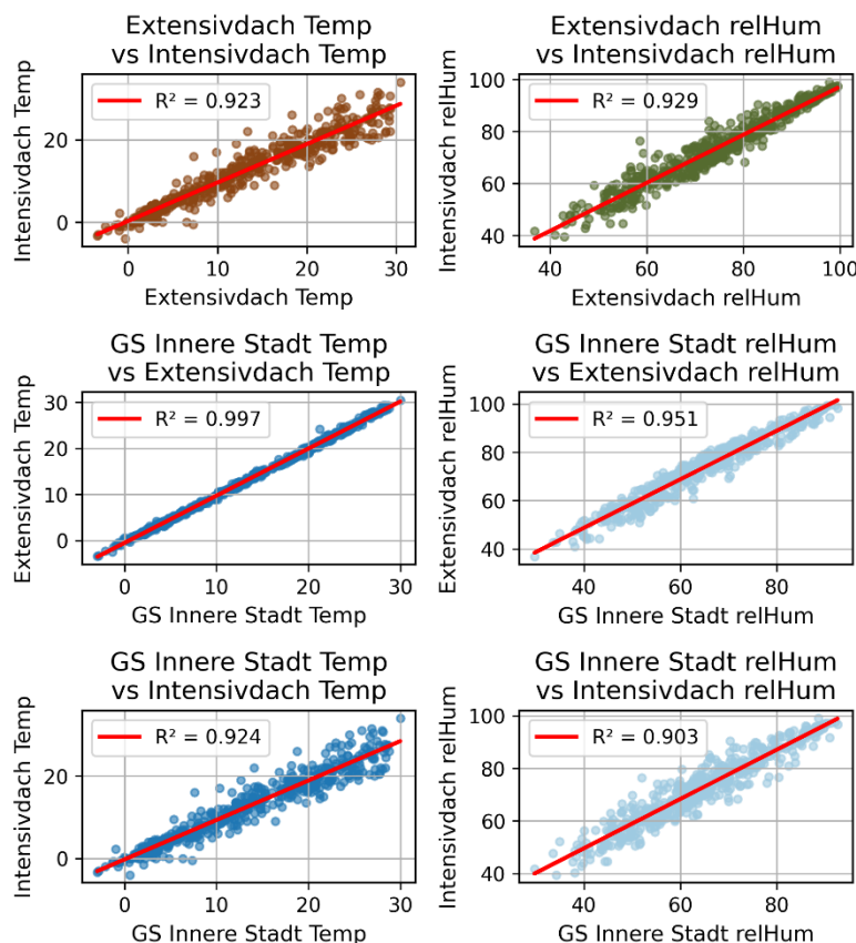
Abbildung 29: Regression von Lufttemperatur und Luftfeuchte am Beispiel Steinbauer Development GmbH, extensiv sowie intensiv [DB1-e und DB1-i] sowie den Messdaten der Geosphere, Wien Innere Stadt (© IBLB).
