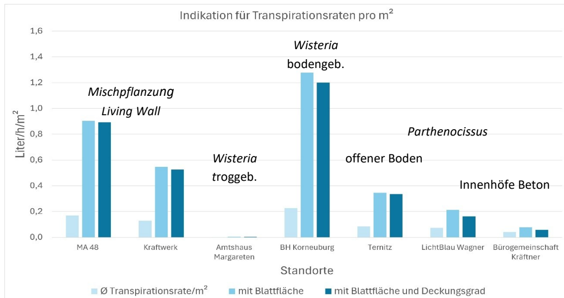
Abbildung 65: Transpirationsraten (2024) für die Fassadenbegrünungen im Vergleich in \text{l/h/m}^2 , sowie hochgerechnet mit LAI und projektivem Deckungsgrad am Quadratmeter (© IBLB).
