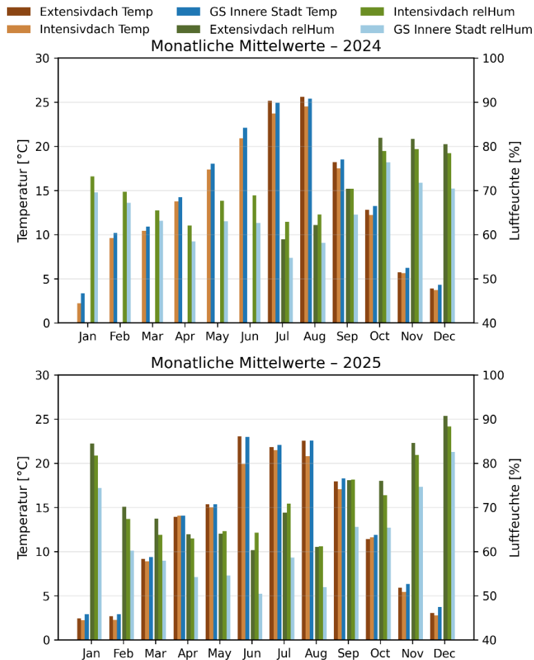
Abbildung 28: Monatliche Gegenüberstellung der mittleren Lufttemperatur beim Messobjekt Steinbauer Development GmbH, extensiv und intensiv [DB1-e und DB1-i] und jener der GeoSphere Austria, Wien Innere Stadt (© IBLB).
