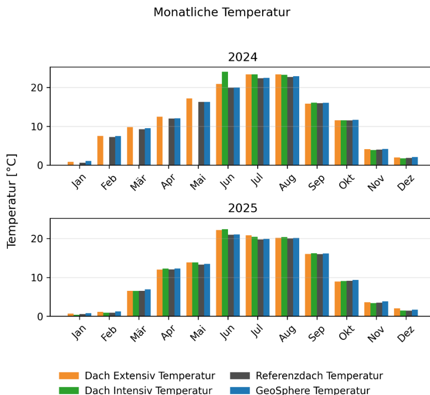
Abbildung 30: Monatliche Gegenüberstellung der mittleren Lufttemperatur beim Messobjekt HTL St. Pölten, extensiv und reduziert-intensiv [DB2-e und DB2-ri] und jener der GeoSphere Austria (© IBLB).
