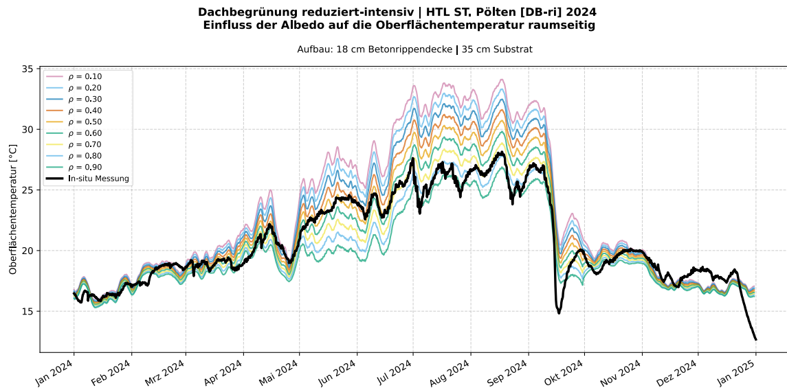
Abbildung 40: Einfluss der Albedo, Simulationsergebnisse; reduziert-intensive Dachbegrünung, HTL St. Pölten [DB2-ri] (© IBO).
