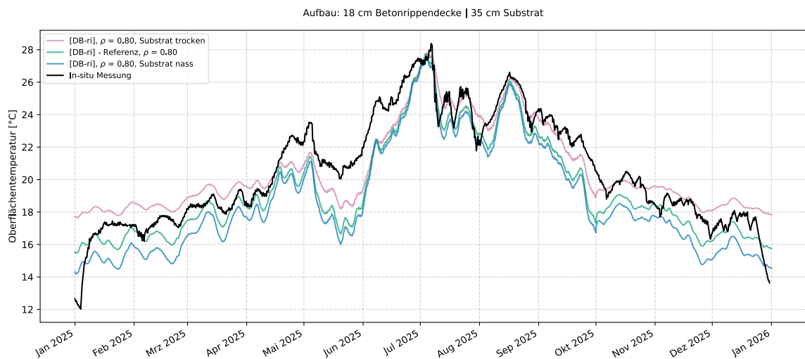
Abbildung 48: Diagramm für 2025: Simulationsergebnisse, Variation Substratfeuchte, Klimadaten 2025; reduziert-intensive Dachbegrünung, HTL St. Pölten [DB2-ri] (© IBO).
