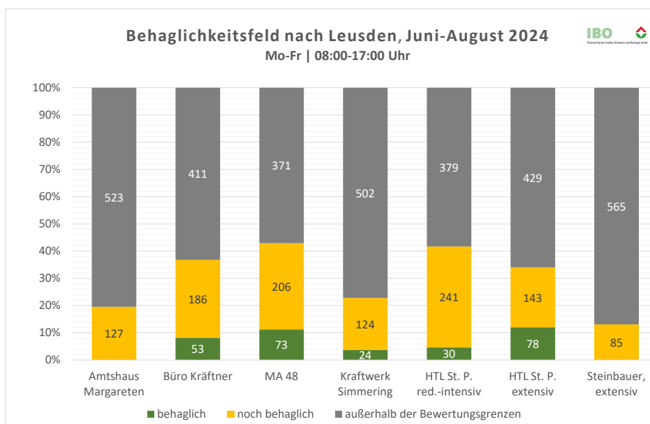
Abbildung 68: Thermische Behaglichkeit nach Freymark und Leusden (1951), alle Dauermessstandorte (© IBO).
