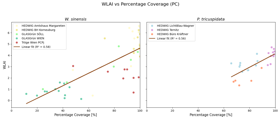
Abbildung 64: Punktwolke und linearer Regressionsfit von WLAI und PC aus dem Datensatz HEDWIG + GLASGrün + TrögeWien (projektiver Deckungsgrad PCPj) für W. sinensis und P. tricuspidata aus HEDWIG (© IBLB).
