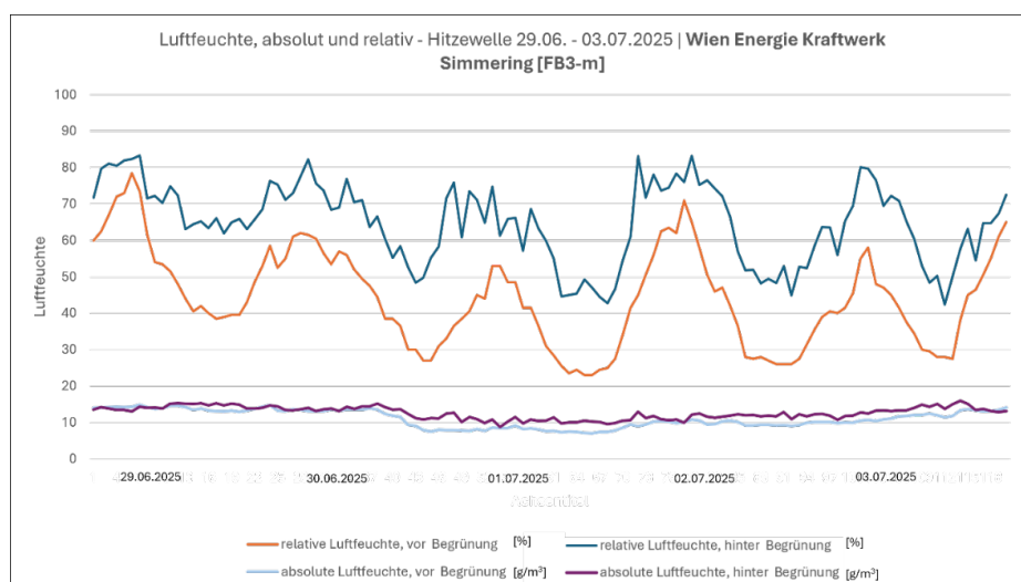
Abbildung 70: Gegenüberstellung Absolute und Relative Luftfeuchte, Hitzewelle 29.06. - 03.07.2025 [Wien Energie Kraftwerk Simmering] (© IBLB).
