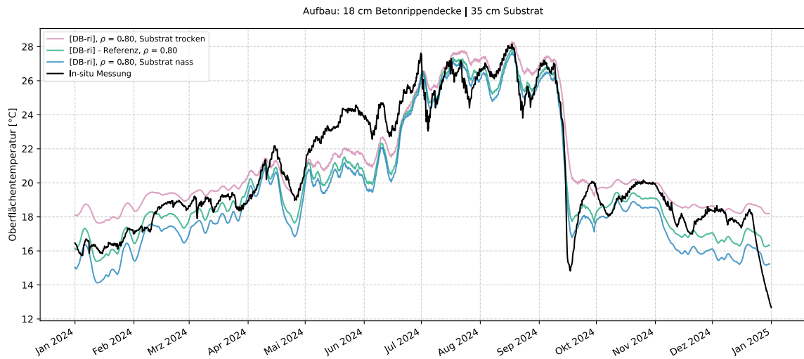
Abbildung 47: Diagramm für 2024: Simulationsergebnisse, Variation Substratfeuchte, Klimadaten 2024; reduziert-intensive Dachbegrünung, HTL St. Pölten [DB2-ri] (© IBO).
