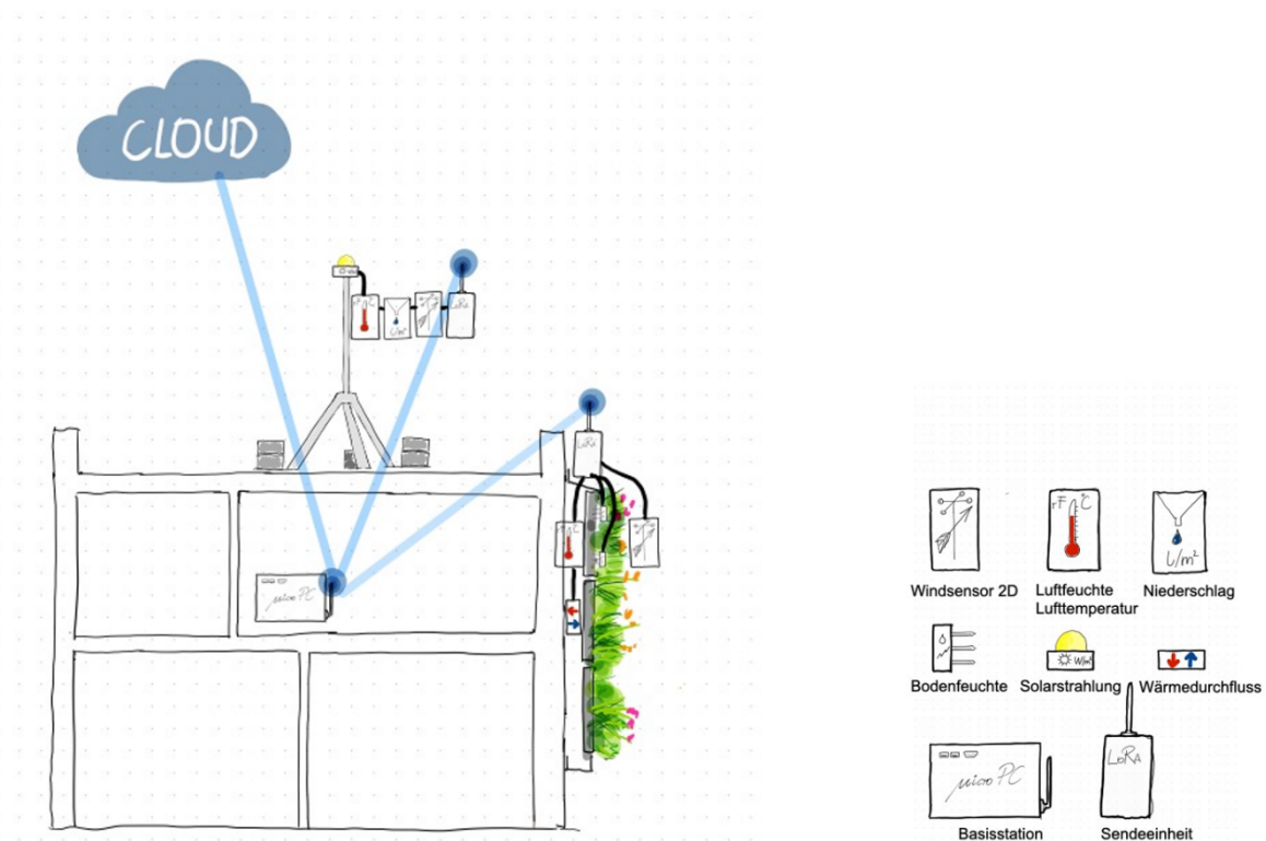
Abbildung 2: Messkonzept Fassadenbegrünungen, Beispiel modulares Begrünungssystem (© IBLB).
