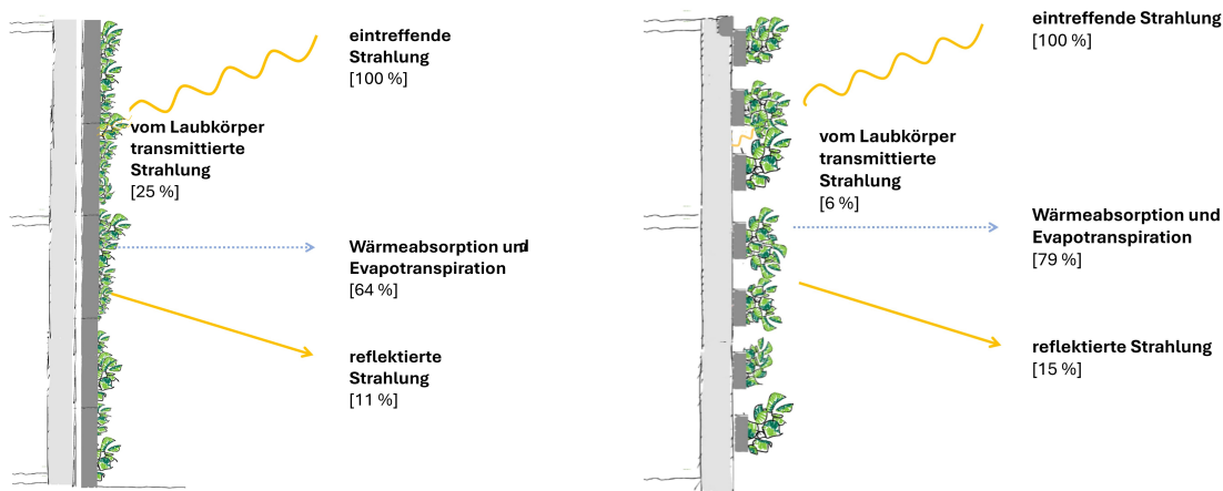
Abbildung 72: kurzwellige Strahlungsbilanz als Mittelwert der in 2024 untersuchten modularen und wandgebundenen Begrünungsobjekte (© IBLB).
