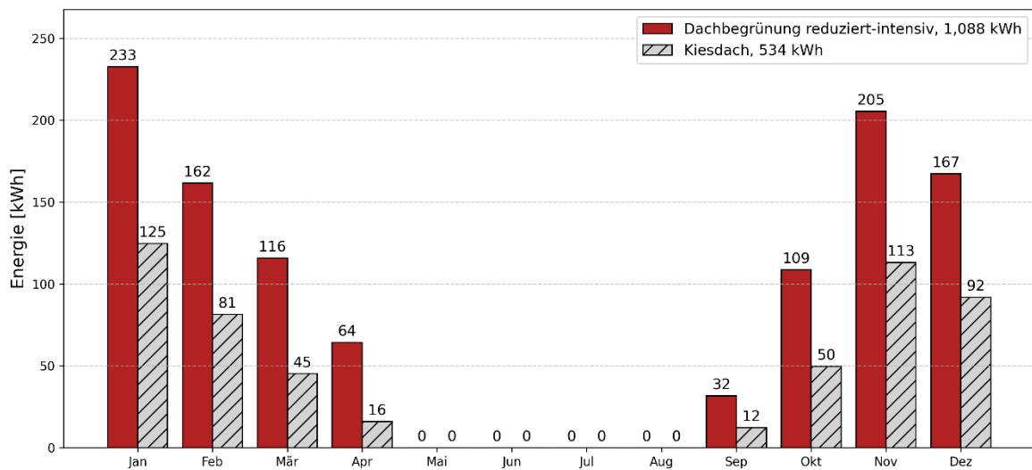
Abbildung 45: Simulationsergebnisse monatlicher Heizenergiebedarf; reduziert-intensive Dachbegrünung (ohne Dämmung) im Vergleich zur Referenz (gedämmtes Kiesdach), HTL St. Pölten [DB2-ri] (© IBO).
