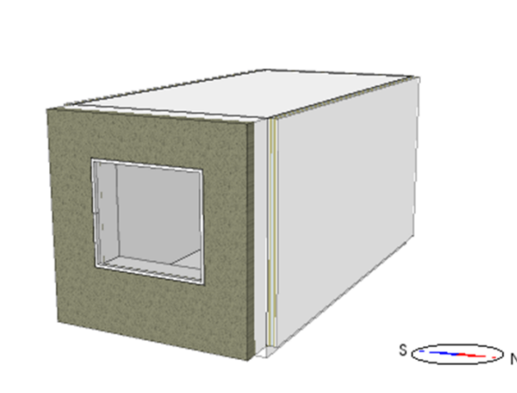
Abbildung 39: links: Simulationsmodell Zone 1, rechts: reduziert-intensive Dachbegrünung, HTL St. Pölten [DB2-ri] (© IBO).
