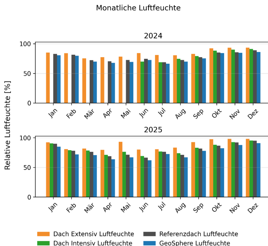
Abbildung 31: Monatliche Gegenüberstellung der mittleren relativen Luftfeuchte beim Messobjekt HTL St. Pölten, extensiv und reduziert-intensiv [DB2-e und DB2-ri] und jener der GeoSphere Austria (© IBLB).
