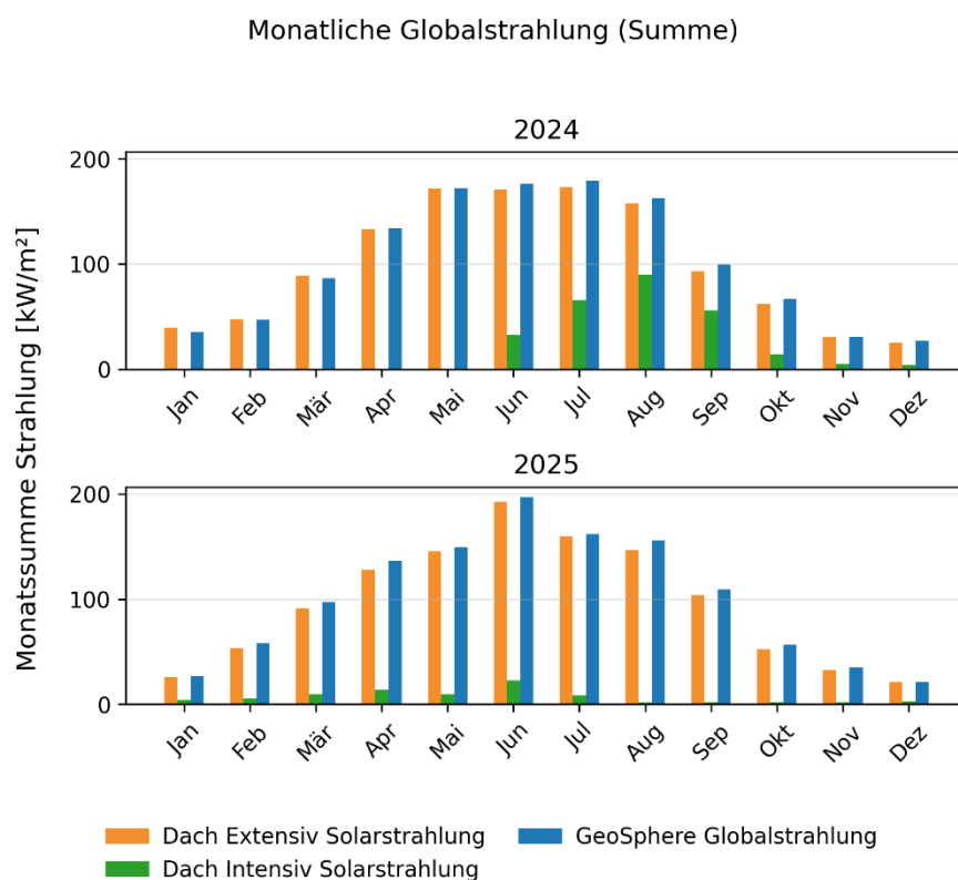
Abbildung 32: Monatliche Gegenüberstellung der mittleren Solarstrahlung beim Messobjekt HTL St. Pölten, extensiv und reduziert-intensiv [DB2-e und DB2-ri] und jener der GeoSphere Austria (© IBLB).
