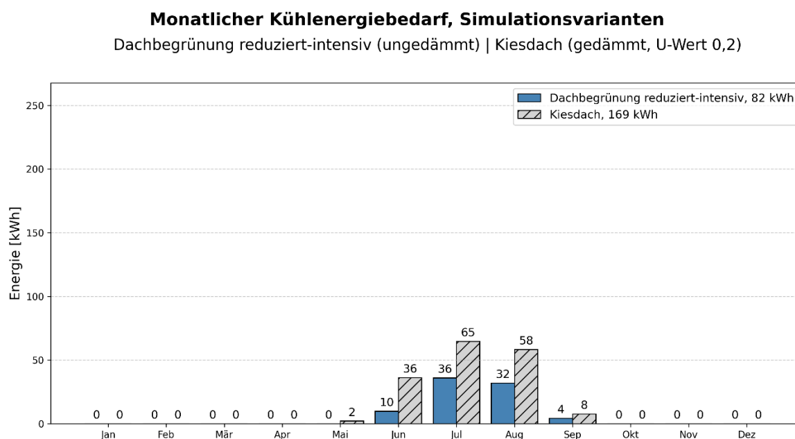
Abbildung 44: Simulationsergebnisse monatlicher Kühlenergiebedarf; reduziert-intensiv Dachbegrünung (ohne Dämmung) im Vergleich zur Referenz gedämmtes Kiesdach HTL St. Pölten [DB2-ri] (© IBO).
