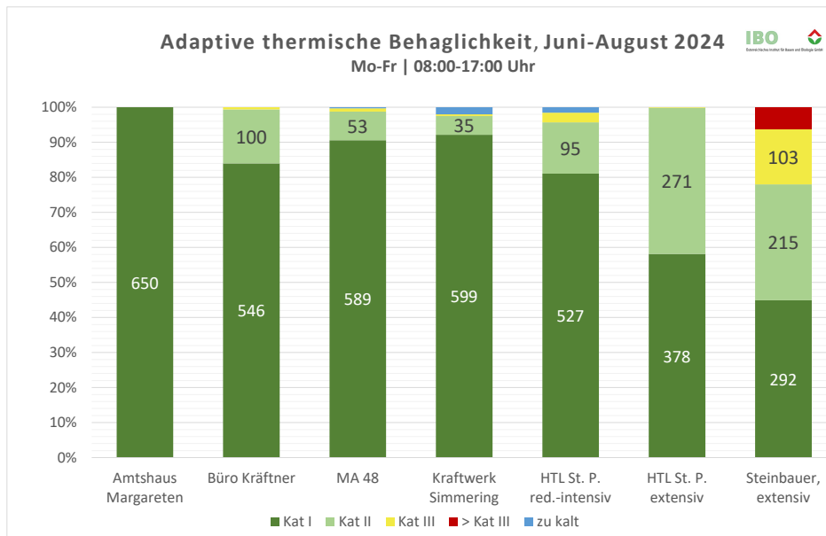
Abbildung 67: Adaptive thermische Behaglichkeit nach ÖNORM EN 16798-1, alle Dauermessstandorte (FB1-tW, FB2-bP, FB3-m, FB4-w, DB1-e, DB1-i, DB2-e, DB2-ri) (© IBO).
