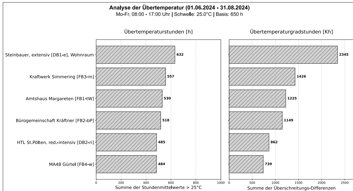
Abbildung 34: Übertemperatur und Übertemperaturgradstunden bei einer Temperaturschwelle von 25°C, Sommer 2024 (© IBO).
