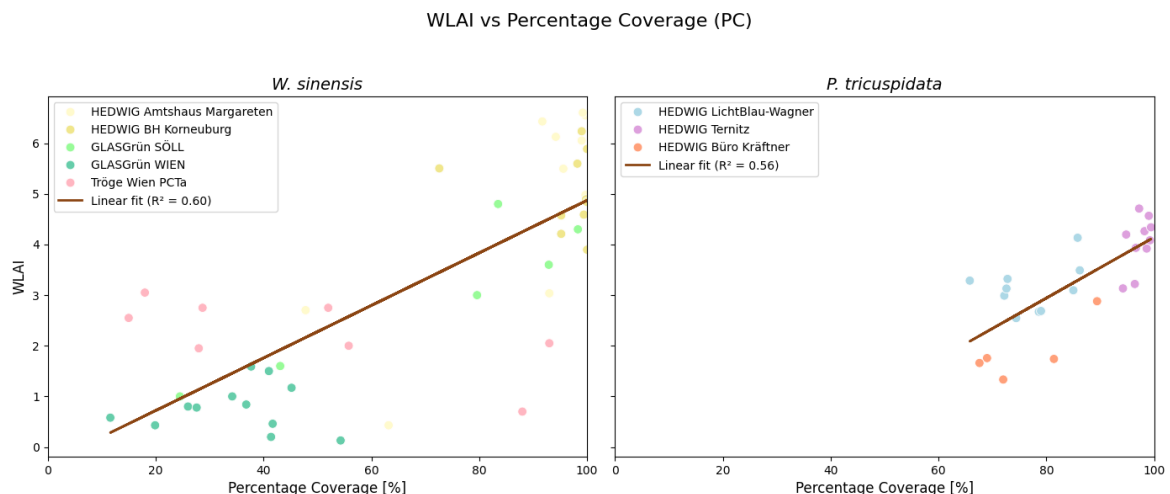
Abbildung 63: Punktwolke und linearer Regressionsfit von WLAI und PC aus dem Datensatz HEDWIG + GLASGrün + TrögeWien (Zieldeckungsgrad PCTa) für W. sinensis und P. tricuspidata aus HEDWIG (© IBLB).
