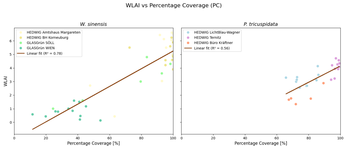
Abbildung 62: Punktwolke und linearer Regressionsfit von WLAI und PC aus dem Datensatz HEDWIG und GLASGrün für W. sinensis und P. tricuspidata aus HEDWIG (© IBLB).
