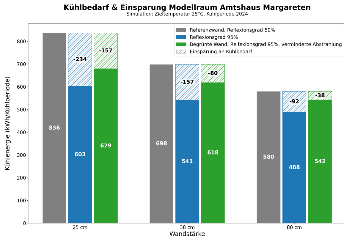
Abbildung 37: Kühlbedarf und Einsparung, Simulationsergebnisse bei unterschiedlichen Wandstärken; Fassadenbegrünung troggebunden, W. sinensis , Amtshaus Margareten [FB1-tW] (© IBO).
