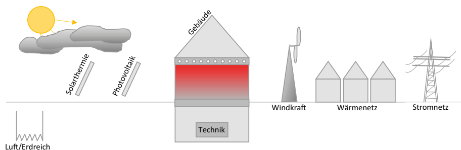
Abb. 14 | 2 Deckung der Wärmeverluste durch gespeicherte Energie (keine Umweltenergie nutzbar)
