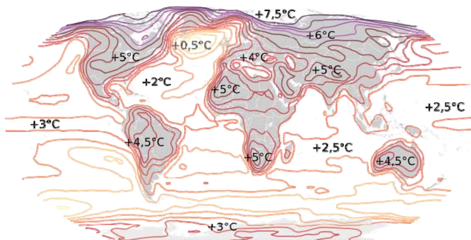
Abbildung 9: Erwärmung von 1980-1999 bis 2090-2099 gemäß dem A1B-Szenario der IPCC (IPCC 2007)
