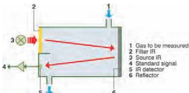
↑ Illustration 98 : Sonde CO2 - procédé photométrique
