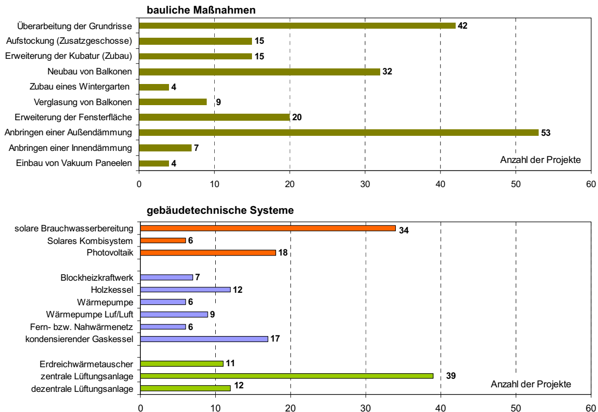
Fig. 7: Auswertung der ausgewählten Demonstrationsgebäude nach baulichen Sanierungsmaßnahmen und nach Verwendung gebäudetechnischer Systeme (Datenquelle: Robert Hastings)
