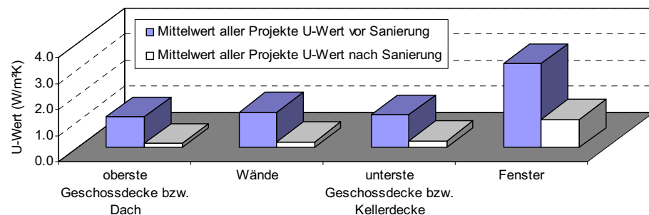
Fig. 8: Auswertung des Wärmeschutzes der Gebäudehüllen (Datenquelle: Robert Hastings)
