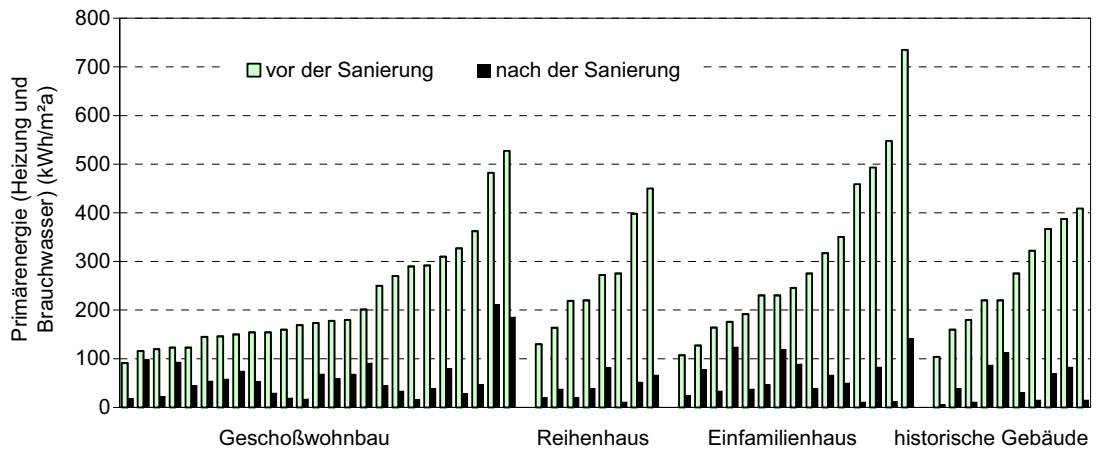
Fig. 9: Primärenergiebedarf für Heizung und Brauchwasser „vor der Sanierung“ im Vergleich zu „nach der Sanierung“ (Datenquelle: Robert Hastings)
