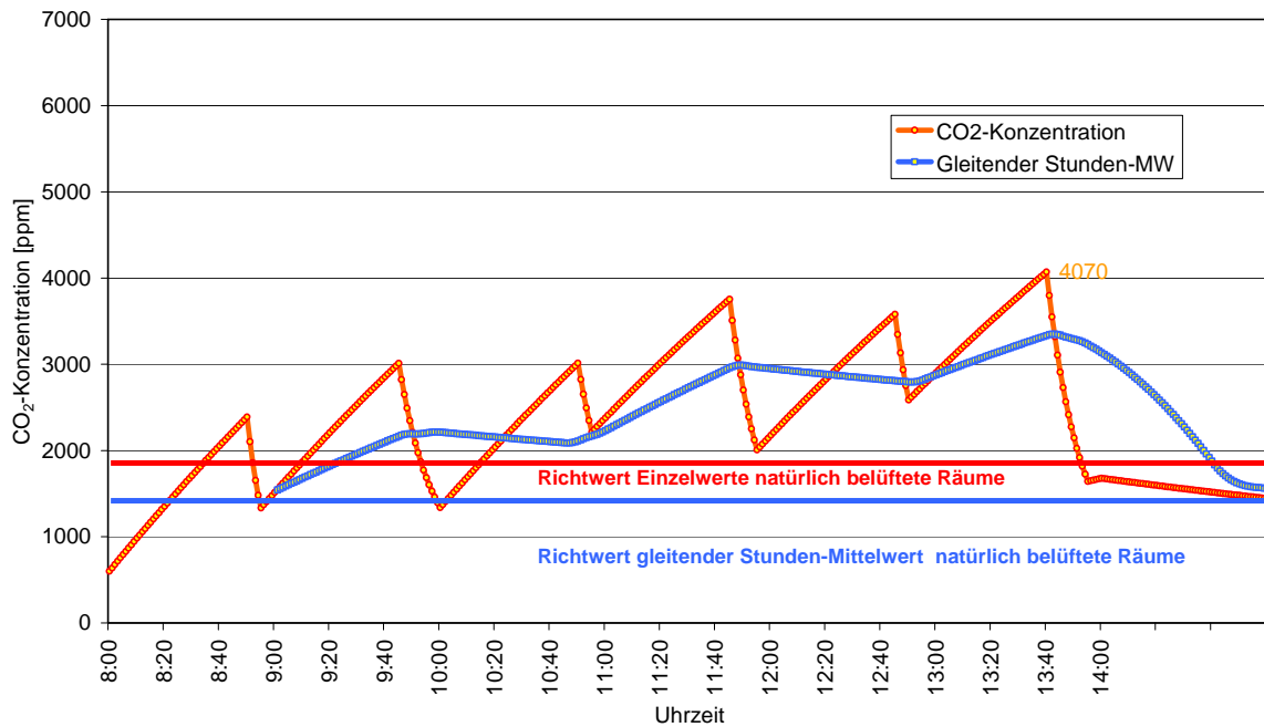
Abbildung 5.13: Gekippte Fenster in der Pause (Querlüftung, 5-facher LW), Land mit 380 ppm CO 2
