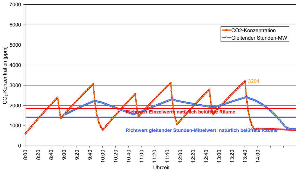
Abbildung 5.14: Ganz geöffnete Fenster in der Pause (10-facher LW), Stadt mit 450 ppm CO 2
