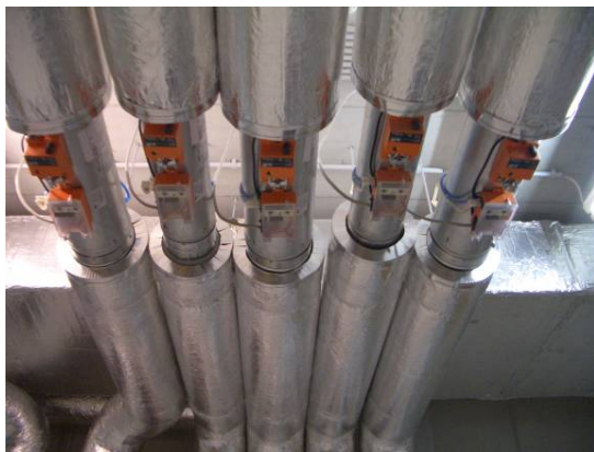
Abbildung 156: Elektrische Stellklappen
