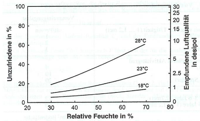
Abbildung 5.4: Der Einfluss von Temperatur und Feuchte auf die empfundene Qualität reiner Luft. (Recknagel et al. 2007/2008)
