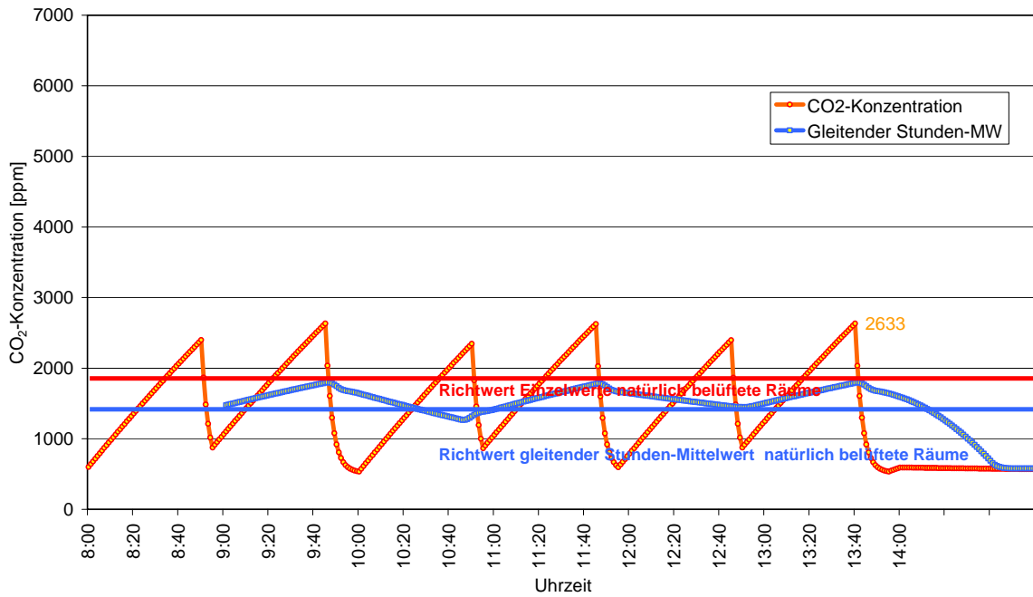
Abbildung 5.15: Ganz geöffnete Fenster in der Pause mit Querlüftungsmöglichkeit (20-facher LW), Stadt mit 450 ppm CO 2
