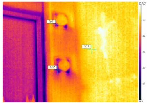
Abbildung 77: Thermographieaufnahme Zuluft t_{\min} = 19,7^{\circ}\text{C}
