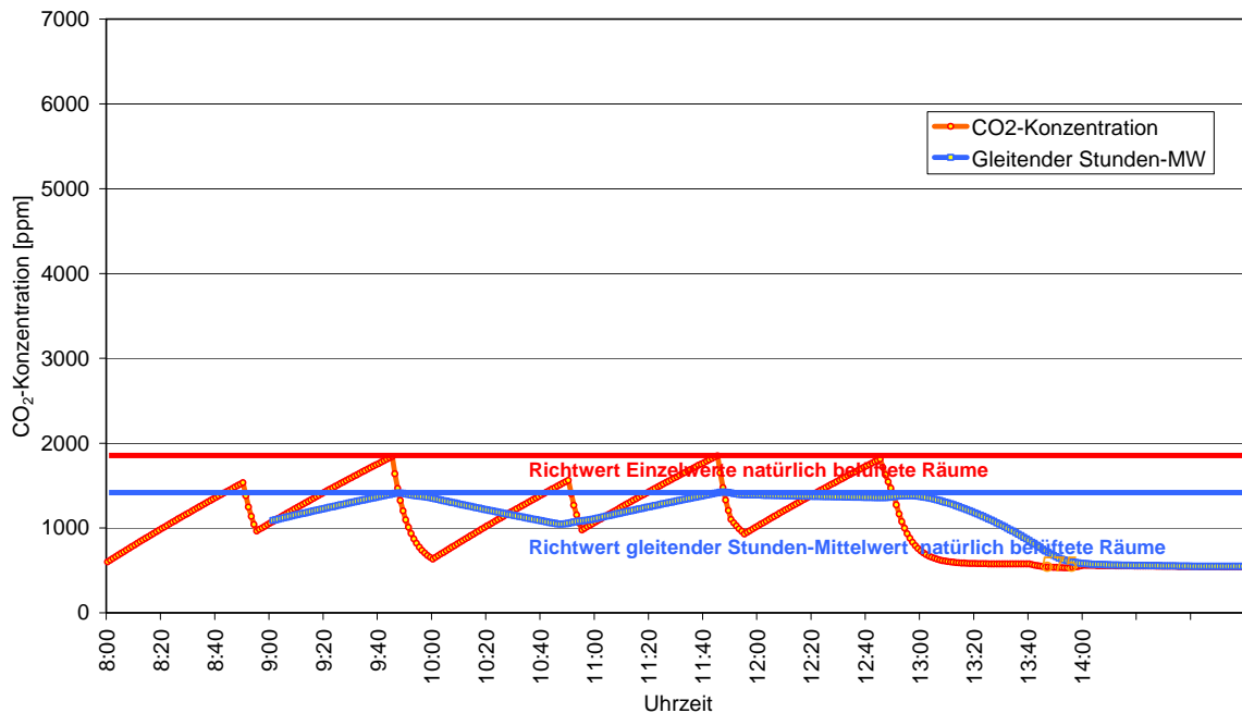
Abbildung 5.17: 360 m 3 Raumvolumen, ganz geöffnete Fenster in der Pause (10-facher LW), Stadt mit 450 ppm CO 2
