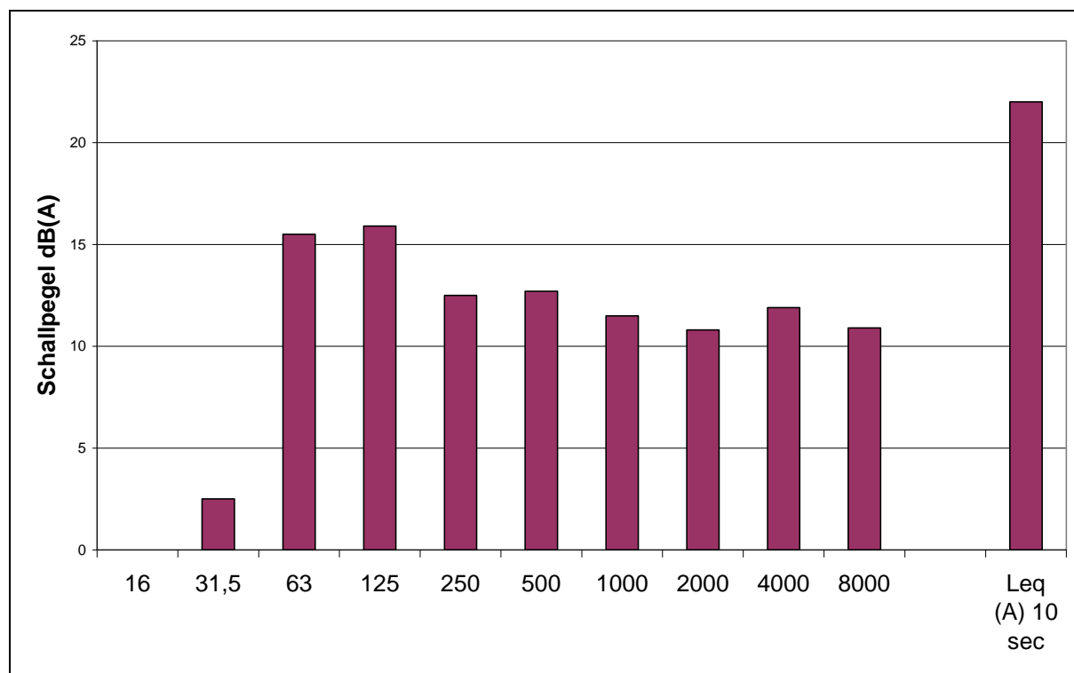
Abbildung 9.15: Frequenzanalyse
