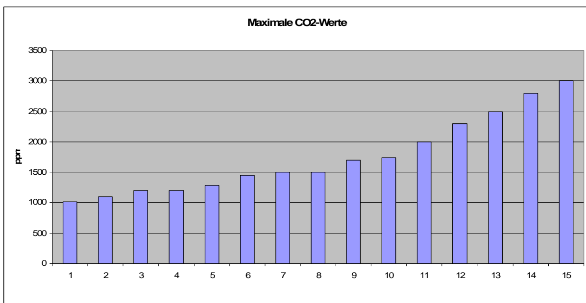
Abbildung 9.21: Maximale CO 2 -Werte in den Klassenzimmern
