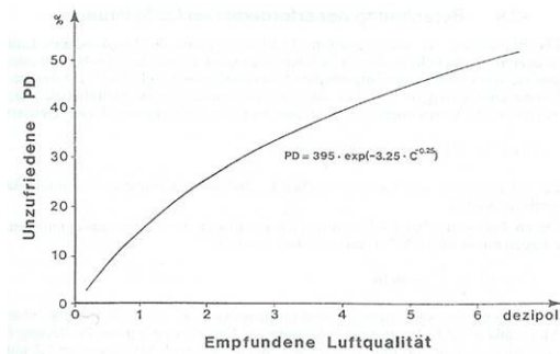
Abbildung 5.6: Abhängigkeit des Geruchspegels und der Unzufriedenheit. (Rechnagel 01/02)
