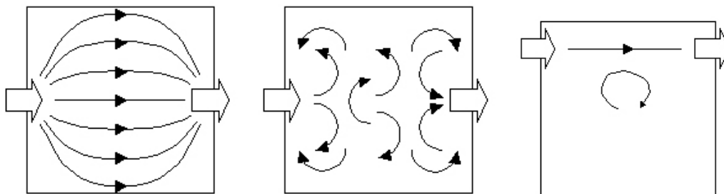
Abbildung 6.15: Verdrängungslüftung – Verdünnungslüftung – Kurzschlusslüftung (Wikipedia – Freie Enzyklopädie)
