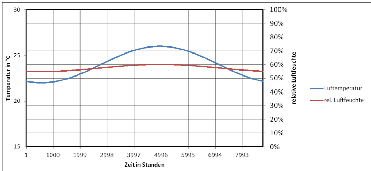
Abbildung 43: Innenraumklima 2 (55 % rel. LF im Winter, basierend auf [OEN03]) – Lufttemperatur und relative Luftfeuchte, Jänner - Dezember
