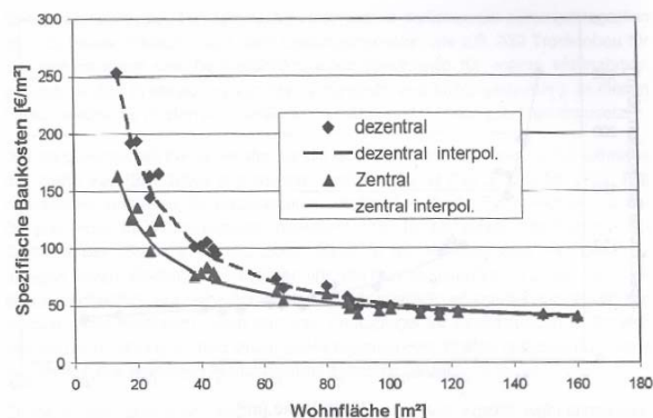
Abbildung 10: Abhängigkeit der Baukosten (netto) von der Wohnfläche der versorgten Wohneinheit; ermittelt anhand von Beispielfgrundrissen; Anlagentyp zentral (8 WE, je zwei WE pro Etage) bzw. dezentral (je ein Gerät pro WE)
