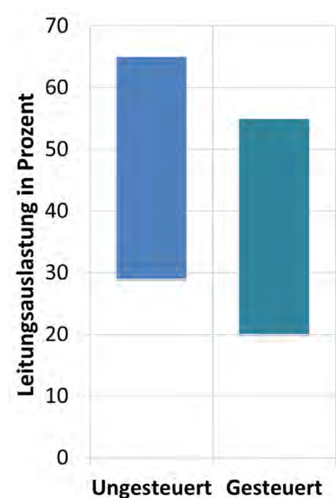
Abb.3: Max. Auslastungen eines Beispielnetzes
