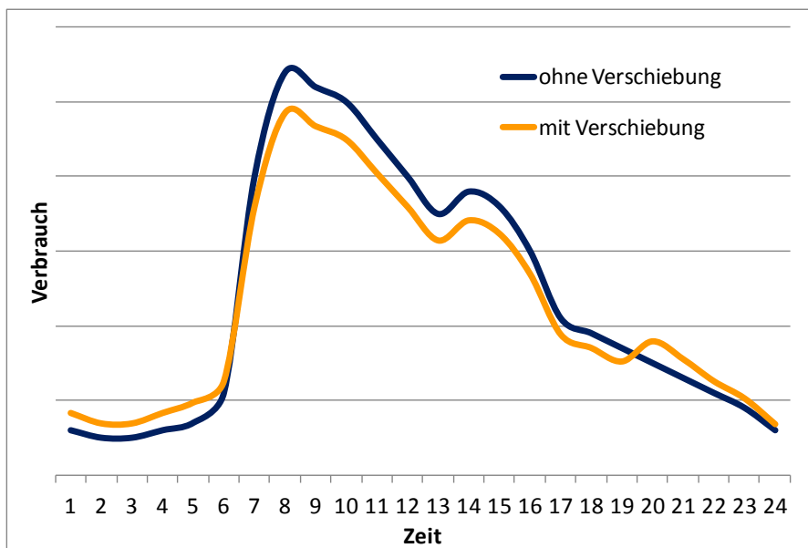
Abbildung 20: Nachfrageverschiebung Business day (beispielhaft)
