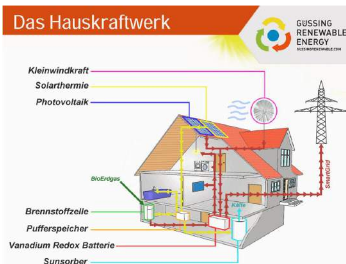
Abbildung 12: Konzept Hauskraftwerk von Güssing Renewable Energy
