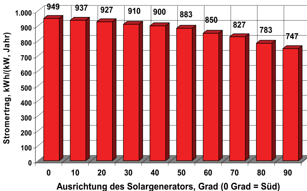
Abb. 17c: Stromertrag einer 3-kW PV-Anlage: Simulation, in Abhängigkeit von der Ausrichtung des Solargenerators
