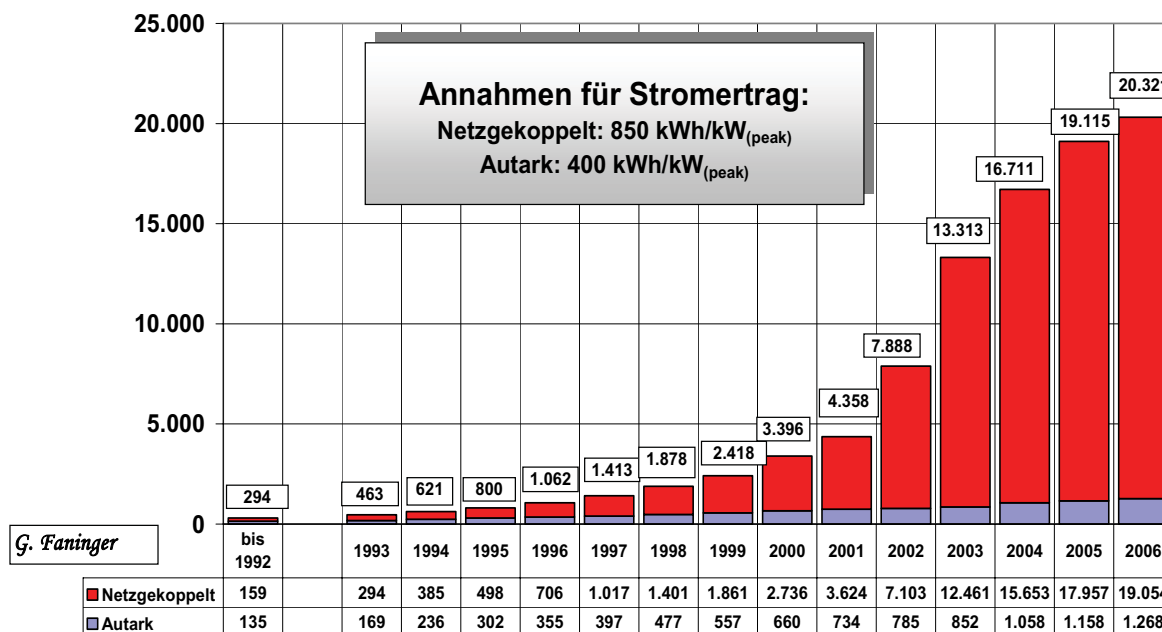
Abb. 20b: Stromertrag von Photovoltaikanlagen in Österreich: 1992 – 2006 Durchschnittliche Voraussetzungen
