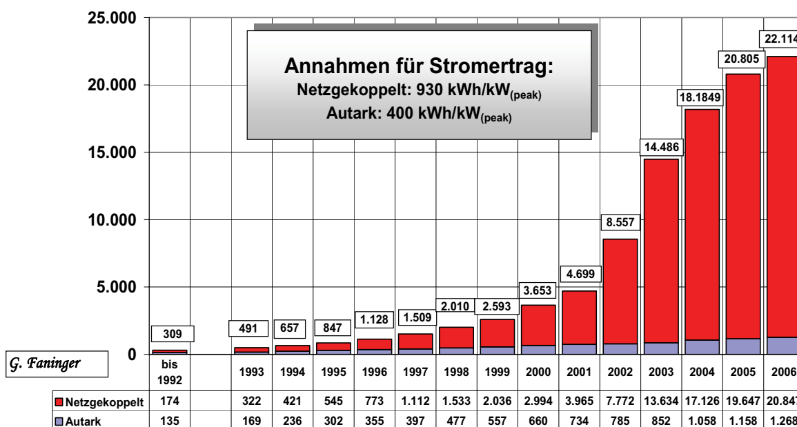
Abb. 20a: Stromertrag von Photovoltaikanlagen in Österreich: 1992 – 2006 Optimale Voraussetzungen
