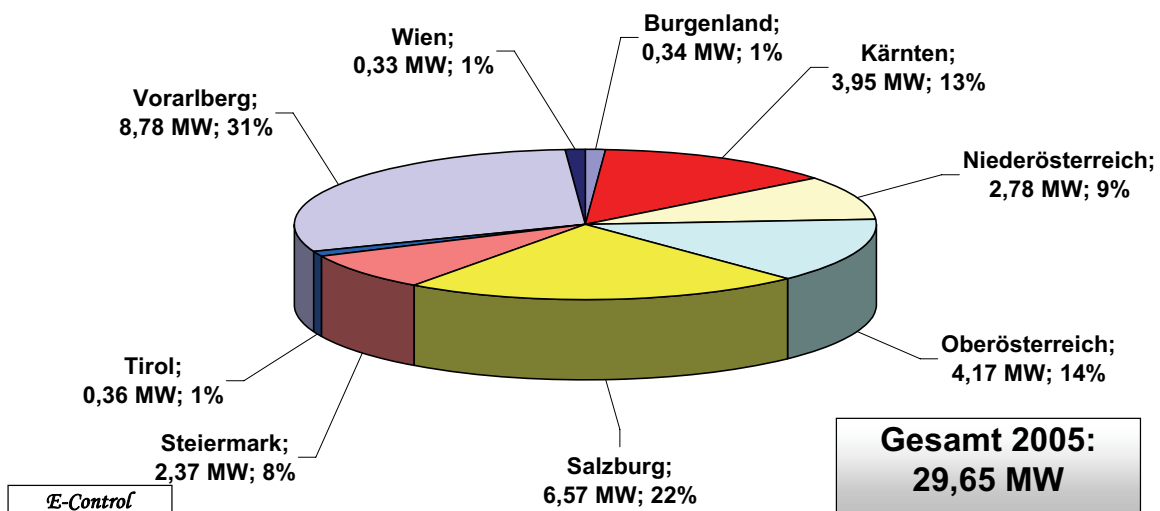
Abb. 15b: Gemäß Ökostromgesetz anerkannte Netzgekoppelte Photovoltaikanlagen: Engpassleistung 2005
