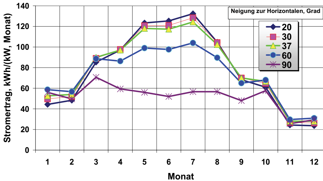
Stromertrag einer Netzgekoppelten Photovoltaikanlage Standort: Klagenfurt, Ausrichtung: Süd
