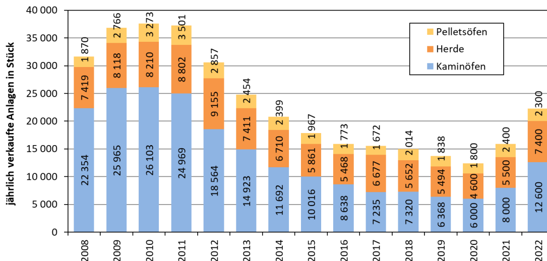
Abbildung 50 – In Österreich verkaufte Biomasseöfen und -herde von 2008 bis 2022 Quelle: BEST (2023)
