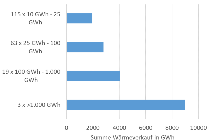
Abbildung 100 – Kategorisierung der 200 größten erhobenen Wärmenetze auf Basis der verkauften Jahreswärmemenge (Datenbasis: 200 Wärmenetze) Quelle: AEE INTEC (2023)
