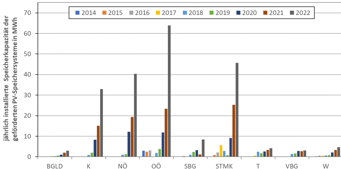
Abbildung 73 – Geförderte und errichtete PV-Speichersysteme je Bundesland Jährlich neu installierte Speicherkapazität der im Rahmen der verfügbaren Förderprogramme errichteten PV-Speichersysteme für die Jahre 2014 bis 2022. Quelle: Technikum Wien (2023)
