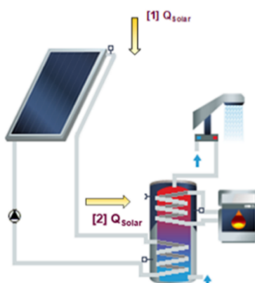
Abbildung 21 – Systemgrenzen bei der Ermittlung der Wärmemengen aus Solarthermie Quelle: AEE INTEC (2023)
