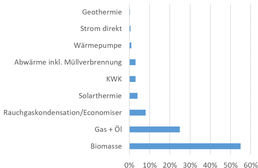
Abbildung 103 – Prozentuelle Verteilung der erhobenen Wärmeerzeugungsanlagen Datenbasis: 1.687 Angaben von 1002 Netzbetreibern Quelle: AEE INTEC (2023)
