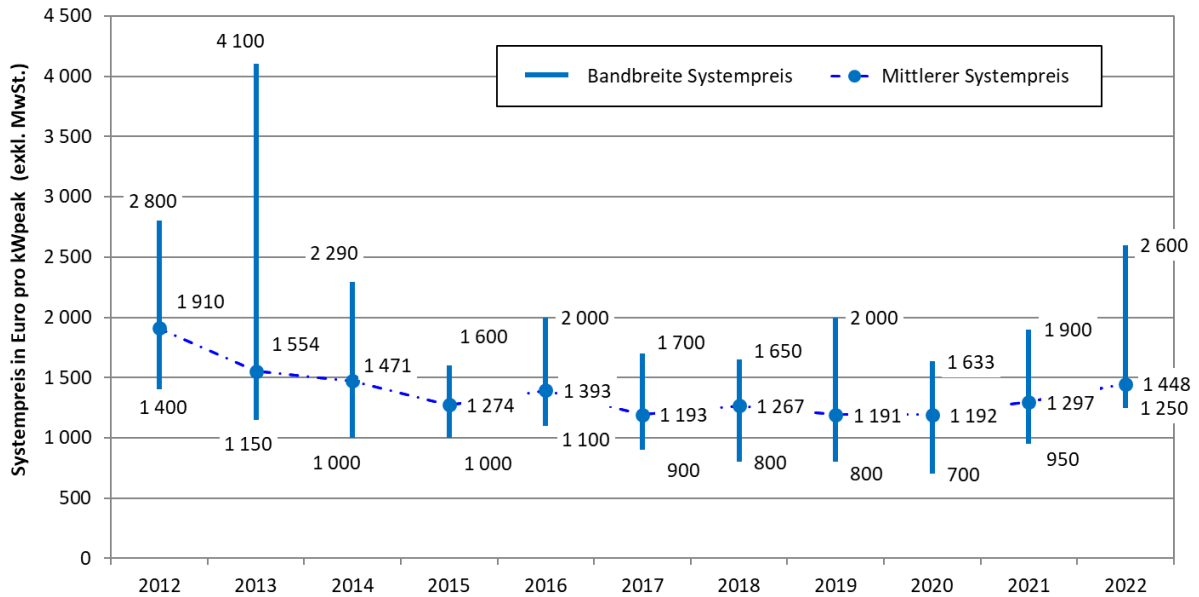
Abbildung 63 – Systempreise für \geq 10 kW peak netzgekoppelte Anlagen 2012 bis 2022 Mittelwert und Bandbreite, fertig installiert, Werte exkl. MwSt.; Anzahl der Nennungen: 2011 n=26, 2012: n=26, 2013: n=28, 2014: n=33, 2015: n=26, 2016: n=20, 2017: n=23, 2018: n=21, 2019: n=23, 2020: n=17, 2021: n=17, 2022: n=13. Quelle: Technikum Wien (2023)
