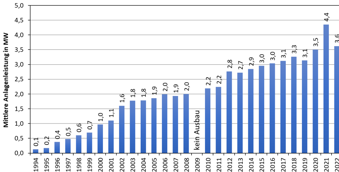
Abbildung 138 – Durchschnittliche Anlagenleistung der Neuinstalltionen Quelle: IG Windkraft (2023)
