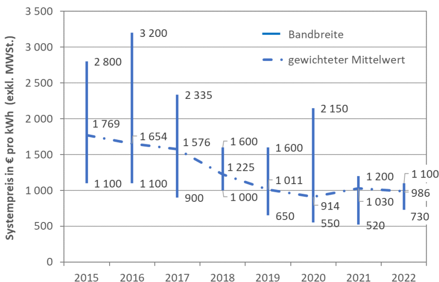
Abbildung 72 – Entwicklung der Systempreise für PV-Speichersysteme in Österreich (Mittelwert und Bandbreite) exkl. MwSt. pro kWh nutzbare Speicherkapazität. Anzahl der Nennungen: 2015: n=9, 2016: n=20, 2017: n=17, 2018: n=10, 2019: n=15, 2020: n = 17, 2021: n = 16, 2022: n = 8. Quelle: Technikum Wien (2023)
