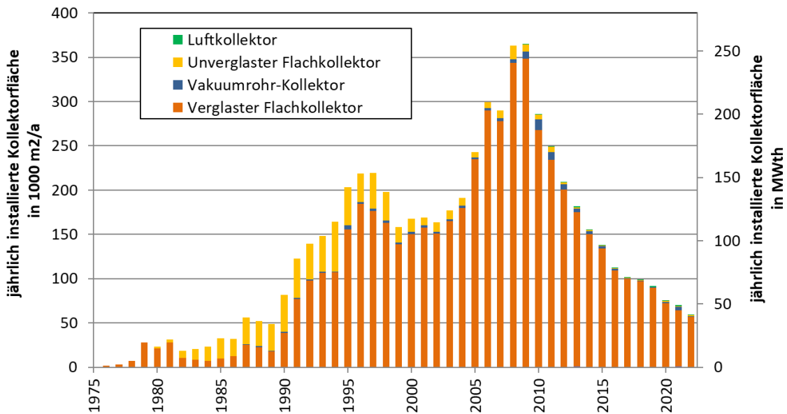
Abbildung 77 – Jährlich installierte Kollektorfläche und Leistung in Österreich von 1975 bis 2022 in m 2 und MW th nach Kollektortyp. Quellen: bis 2006: Faninger (2007), ab 2007: AEE INTEC (2023)
