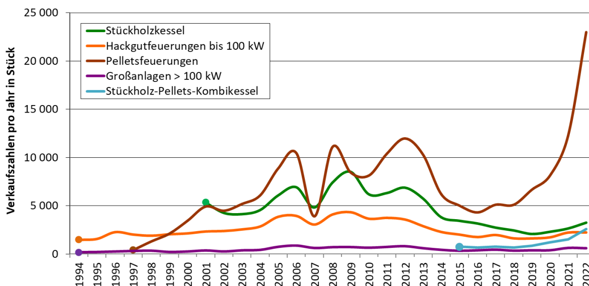
Abbildung 2 – Die Marktentwicklung von Biomassekesseln in Österreich bis 2022
