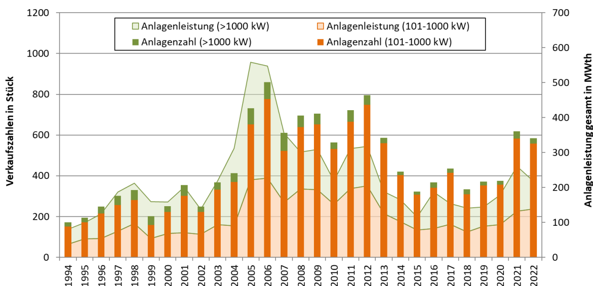
Abbildung 46 – Jährlich in Österreich verkaufte Biomassekessel großer Leistung von 1994 bis 2022. Quelle: LK NÖ (2023)
