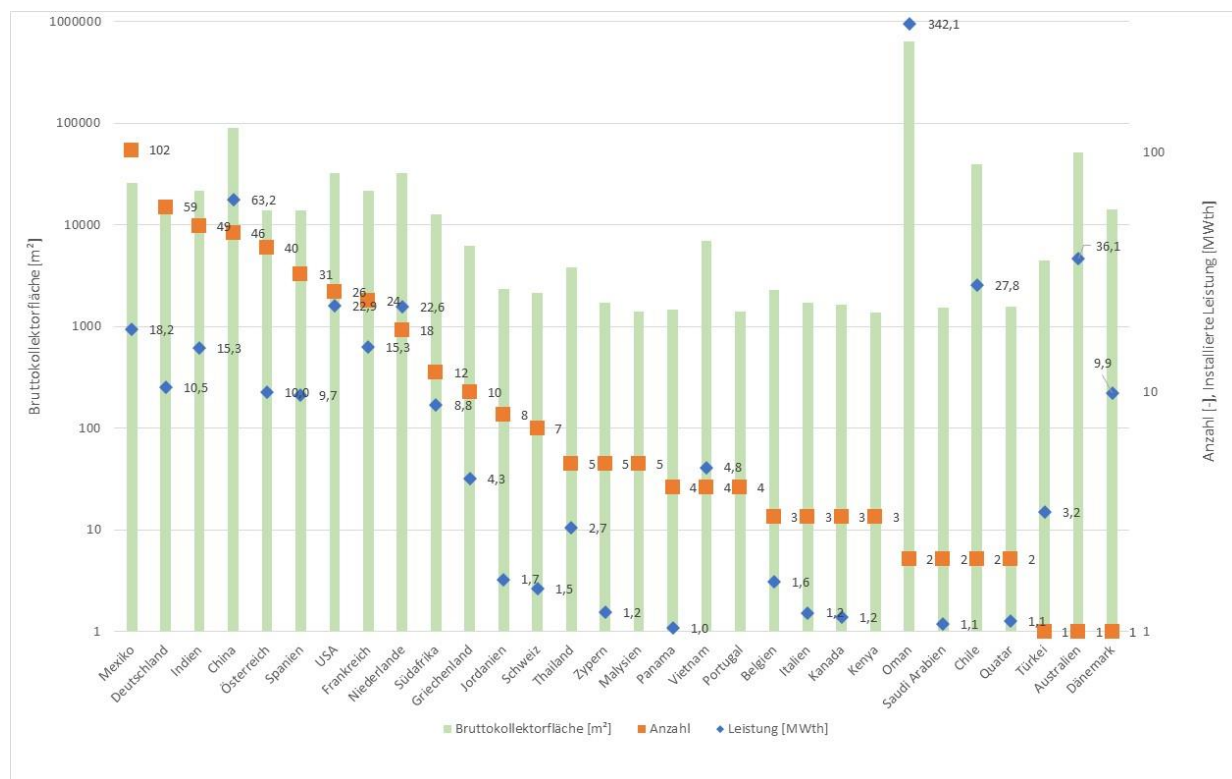
Abbildung 86 – Solare Prozesswärmanlagen weltweit im Jahr 2022 für Länder zu denen Detaildaten vorliegen. Quelle: Weiss, W., Spörk-Dür, M. (2023)
