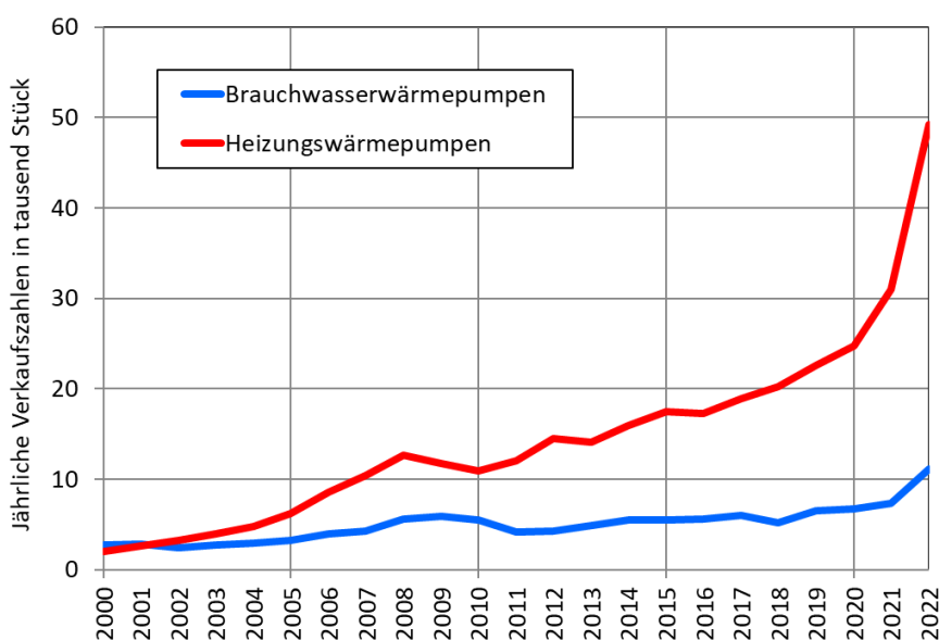
Abbildung 114 – Brauchwasser- und Heizungswärmepumpen in Österreich bis 2022 Quellen: bis 2006: Faninger (2007), ab 2007: Biermayr et al. (2022), ENFOS (2023)
