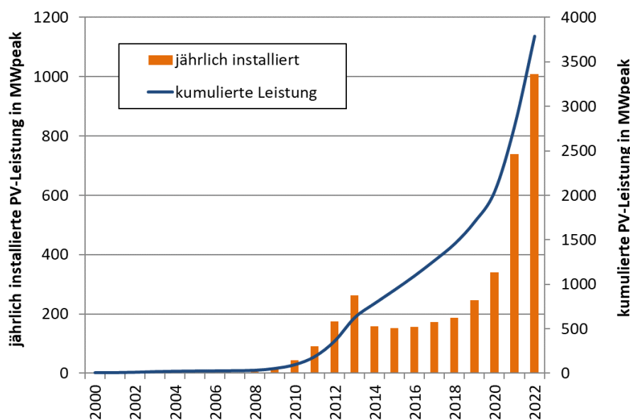
Abbildung 3 – Die Marktentwicklung der Photovoltaik in Österreich bis 2022
