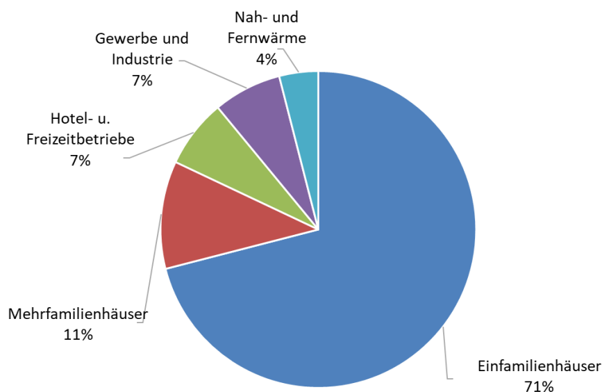
Abbildung 79 – Neu installierte thermische Solaranlagen 2022 nach Einsatzbereichen Quelle: AEE INTEC (2023)
