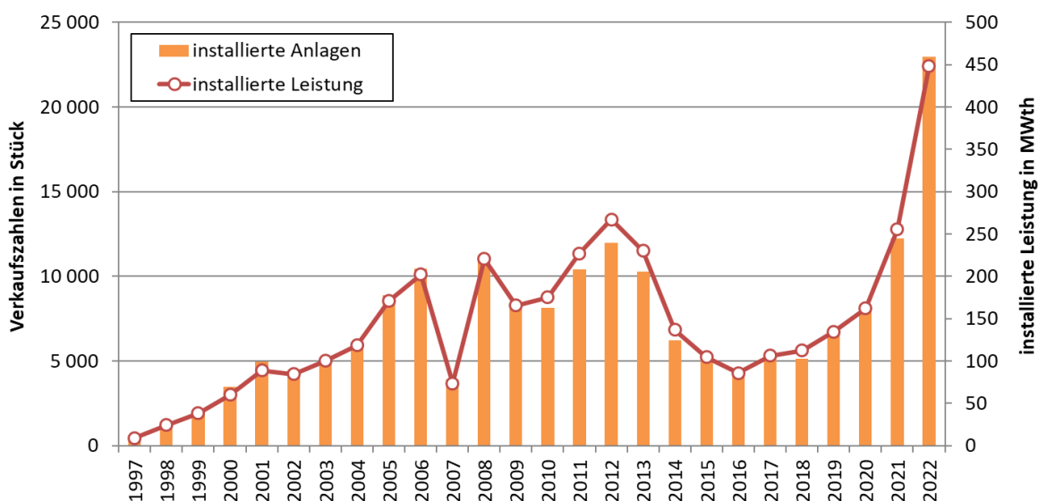
Abbildung 45 – Jährlich installierte Pelletsboiler < 100 kW th in Stück und installierter Leistung in MW th von 1997 bis 2022. Quelle: LK NÖ (2023)
