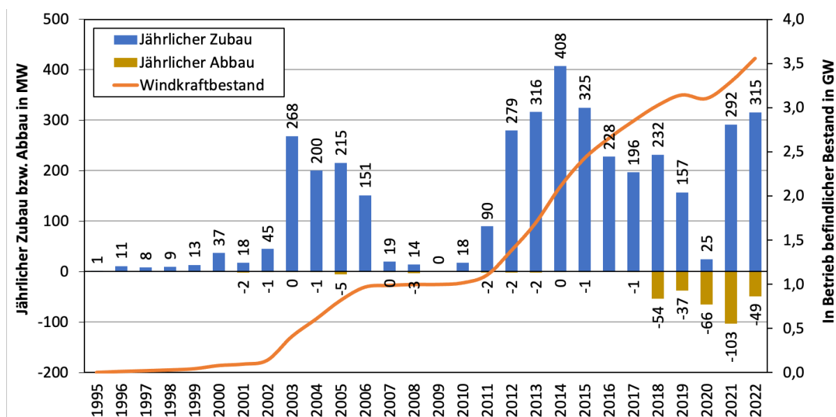
Abbildung 134 – Die Marktentwicklung der Windkraft in Österreich bis 2022
