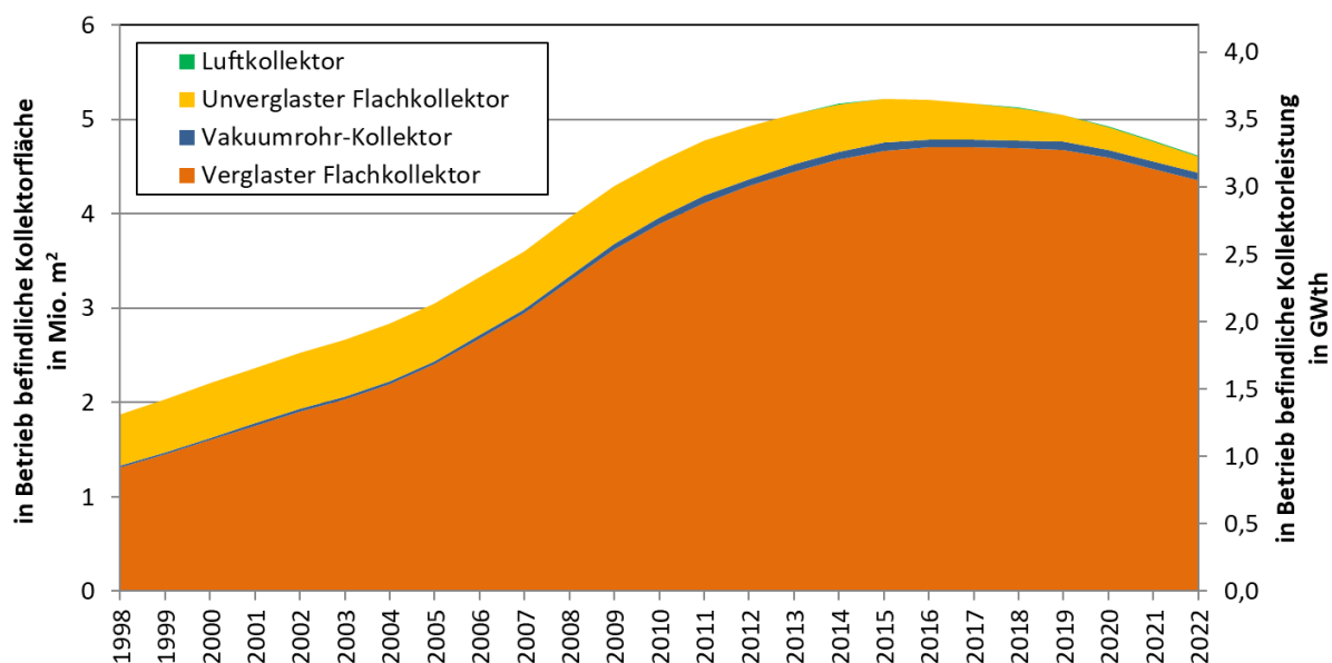
Abbildung 78 – In Betrieb befindliche thermische Kollektoren in Österreich Kollektorfläche bzw. installierte Leistung in den Jahren 1998 bis 2022. Quellen: bis 2006: Faninger (2007), ab 2007: AEE INTEC (2023)
