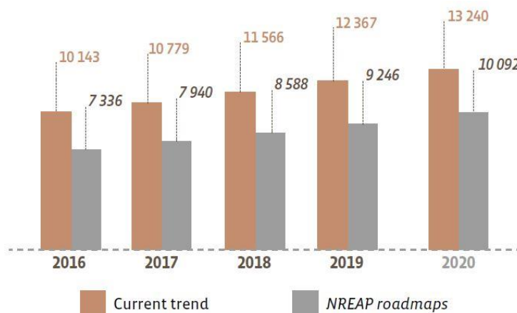
Abbildung 123 – Umweltwärme aus Wärmepumpen in den EU28 in kt Tatsächlicher Trend und Ziele der nationalen Aktionspläne. Quelle und Bildnachweis: Euroobserver (2021)
