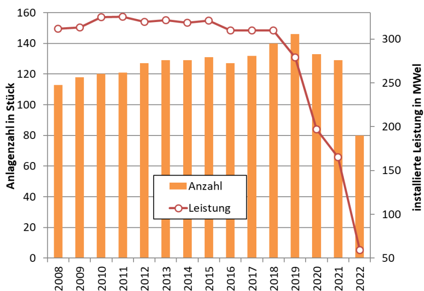
Abbildung 49 – Bestandsentwicklung Ökostromanlagen mit Brennstoff feste Biomasse installierte Leistung aktiver Anlagen in MW el . Datenquelle: OeMAG (2023b)
