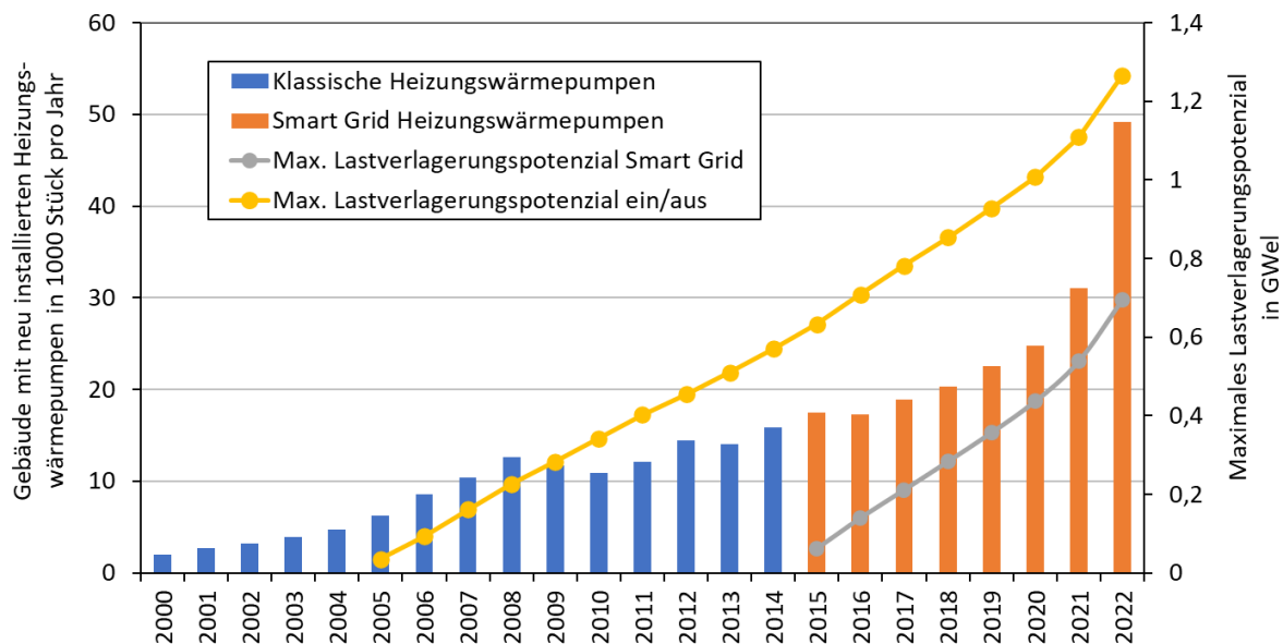
Abbildung 130 – Maximales Lastverlagerungspotenzial von Heizungswärmepumpen in Österreich. Quelle: ENFOS (2023)
