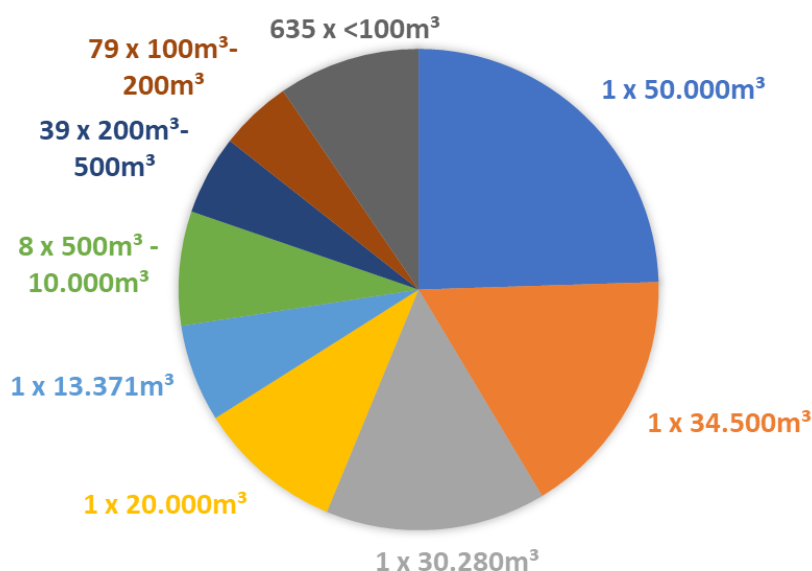
Abbildung 6 – Verteilung des gesamten Behälterspeichervolumens je erhobenem Wärmenetz im Jahr 2022. Datenbasis: 766 Wärmenetze Quelle: AEE INTEC (2023)
