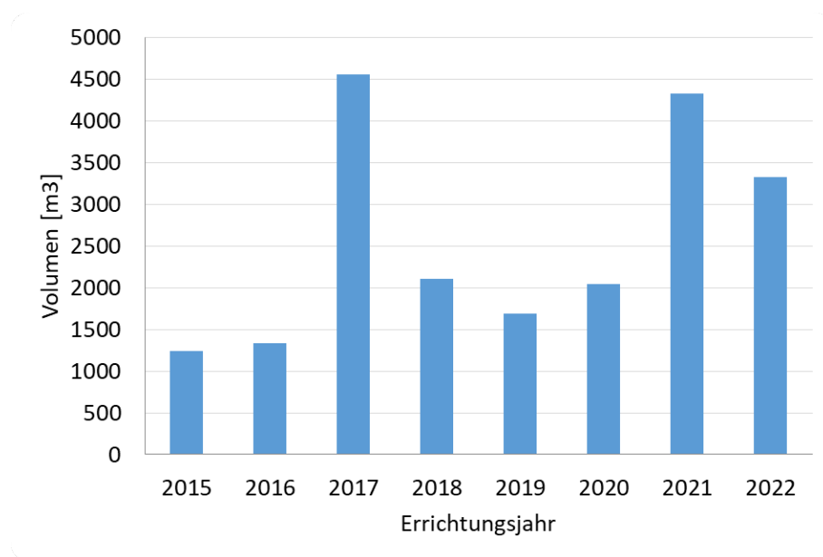
Abbildung 105 – Volumen von Behälterwasserspeichern über Errichtungsjahr von 2015 bis 2022 (Datenbasis: 259 Wärmespeicher in 226 Wärmenetzen) Quelle: AEE INTEC (2023)
