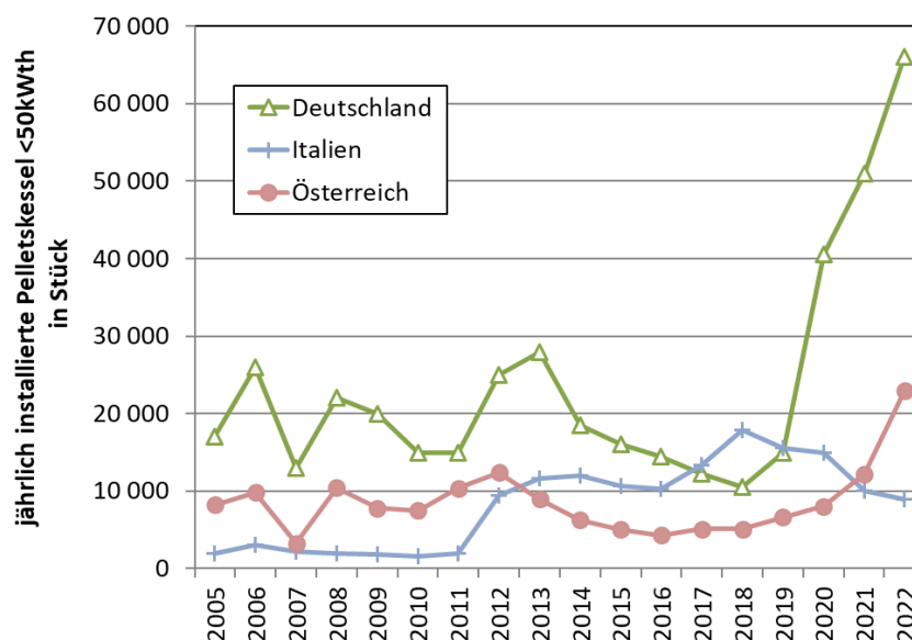
Abbildung 51 – Pelletskessel < 50 kW in Deutschland, Italien und Österreich jährliche Neuinstallationen. Quellen: DEPI (2023), AIEL (2023), LK NÖ (2023a)
