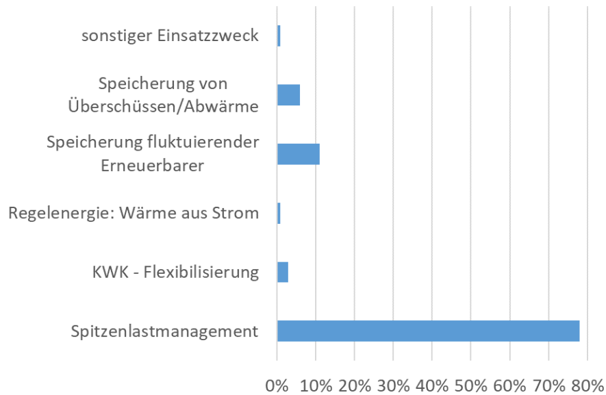
Abbildung 108 – Nutzung der installierten Speicherkapazitäten in den insgesamt erhobenen Wärmenetzen (Datenbasis: 289 Speichernutzungsangaben für 227 Wärmenetze, Mehrfachnennungen je Netz möglich) Quelle: AEE INTEC (2023)
