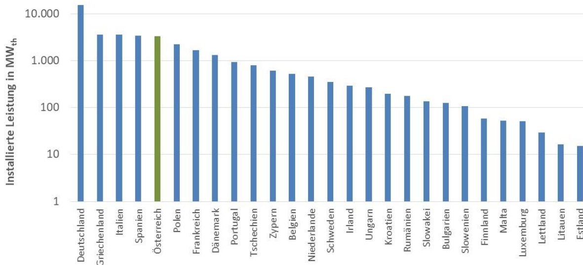
Abbildung 98 – Bestand thermischer Solaranlagen in den EU27 Ländern Datenstand Jänner 2022. Quelle: AEE INTEC (2023)
