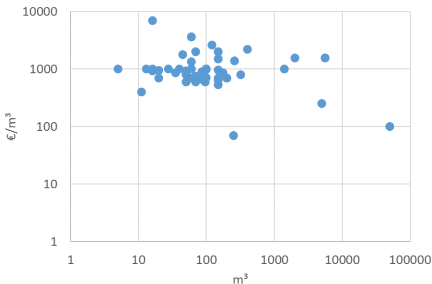
Abbildung 111 – Verteilung der Preisangaben von 59 Behälterwasserspeichern inkl. Kosten für Wärme- und Witterungsschutz sowie anteiliger baulicher Kosten, exkl. Umsatzsteuer (Datenbasis: 59 Wärmespeicher) Quelle: AEE INTEC (2023)
