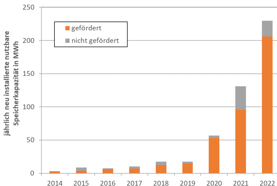
Abbildung 70 – Jährlich neu installierte PV-Batteriespeicher von 2014 bis 2022 in Österreich geförderte und nicht geförderten Systeme.
