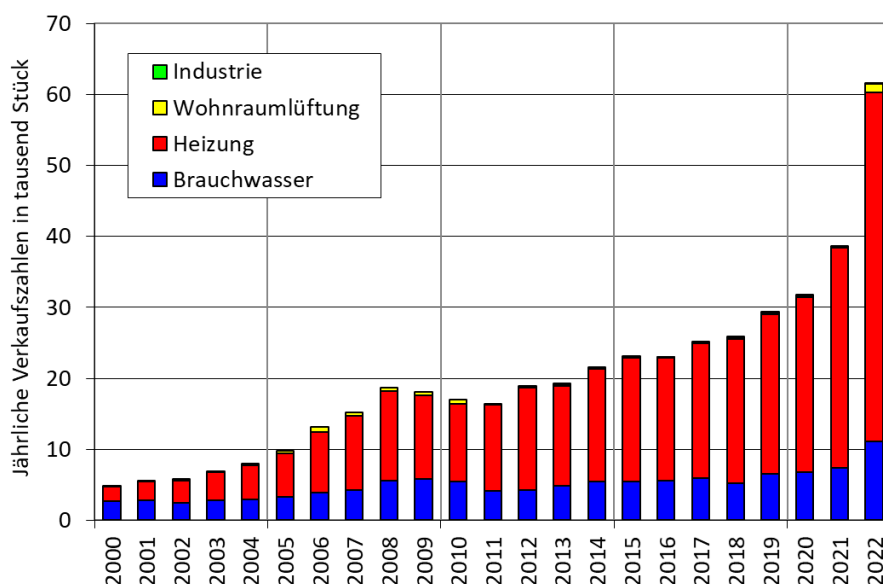
Abbildung 113 – Wärmepumpen-Verkaufszahlen in Österreich bis 2022
