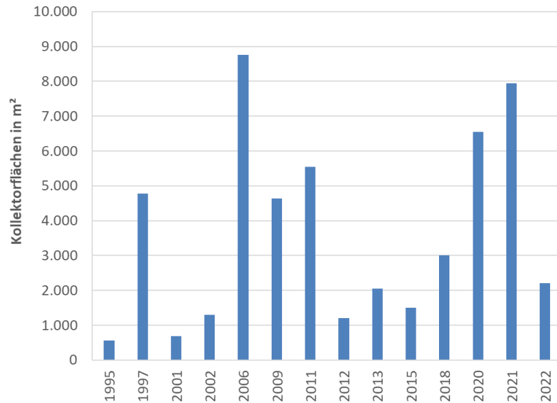
Abbildung 96 – Historischer Verlauf der jährlich neu installierten Solaranlagen für Nah- und Fernwärmenetze. Quelle: AEE INTEC (2023)
