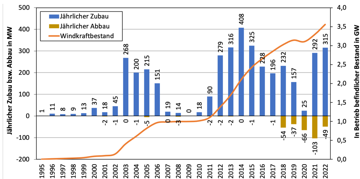
Abbildung 9 – Die Marktentwicklung der Windkraft in Österreich bis 2022
