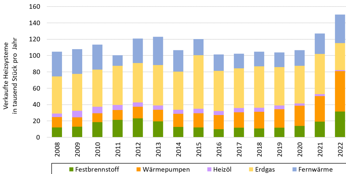
Abbildung 28 – Jährlich in Österreich verkaufte Heizungssysteme von 2008 bis 2022 Quellen: BEST (2023), ENFOS (2023), VÖK (2019), VÖK (2023), Statistik Austria (2023i)
