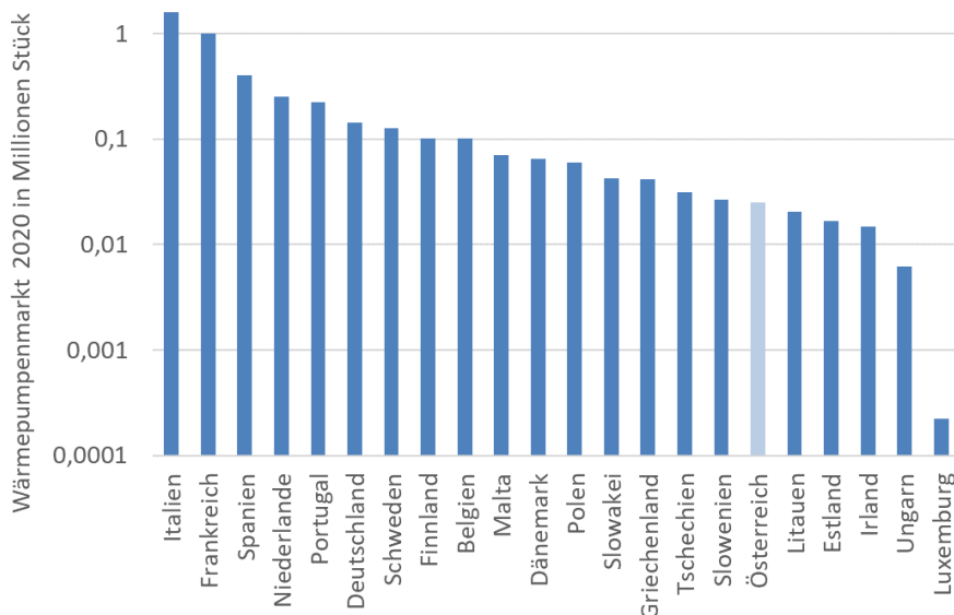
Abbildung 122 – Wärmepumpenmarkt in EU27-Ländern im Jahr 2020 Quelle: Euroobserver (2021)
