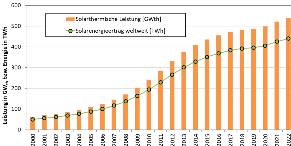
Abbildung 83 – Weltweit installierte Leistung und Energieerträge 2000-2022
