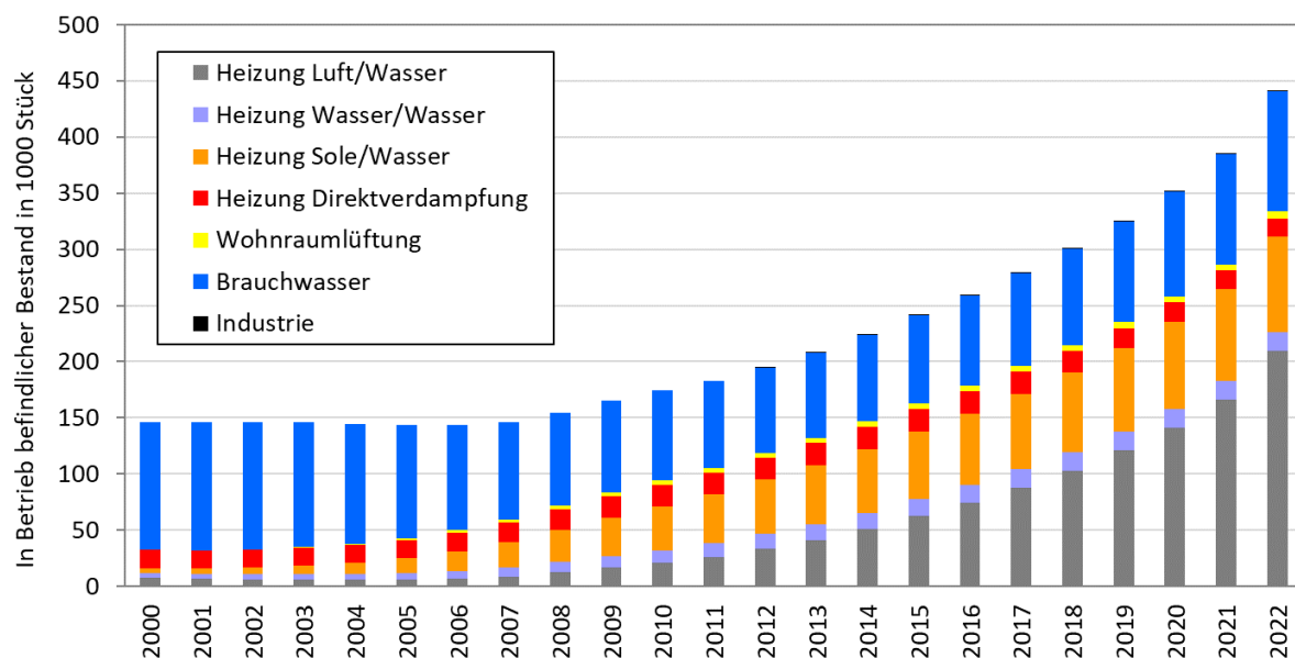
Abbildung 119 – In Betrieb befindlicher Wärmepumpenbestand in Österreich nach Arten und Wärmequellsystemen.
