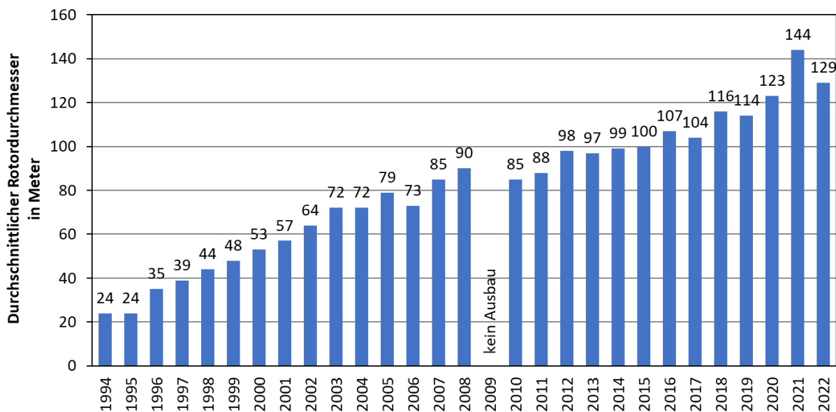
Abbildung 139 – Durchschnittlicher Rotordurchmesser der Neuinstalltionen Quelle: IG Windkraft (2023)
