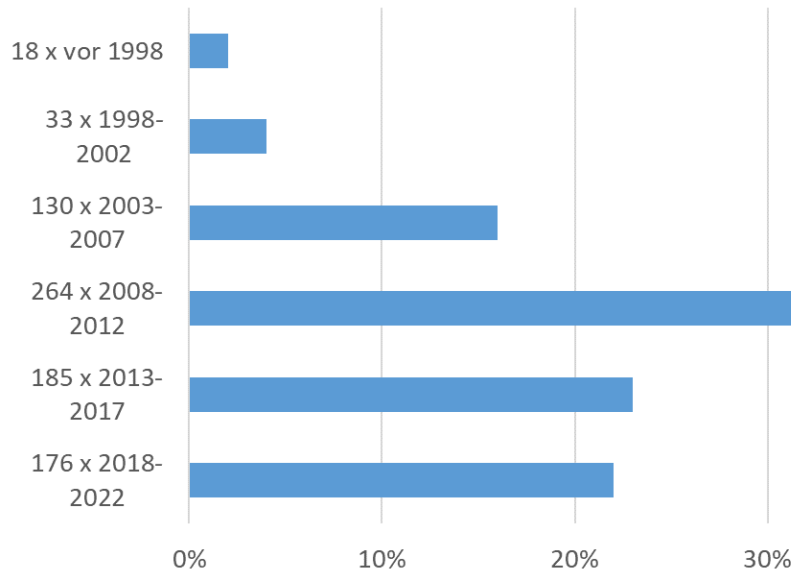
Abbildung 104 – Prozentuelle Verteilung der Speichererrichtungsjahre für Behälterwasserspeicher (Datenbasis: 608 Wärmenetze) Quelle: AEE INTEC (2023)
