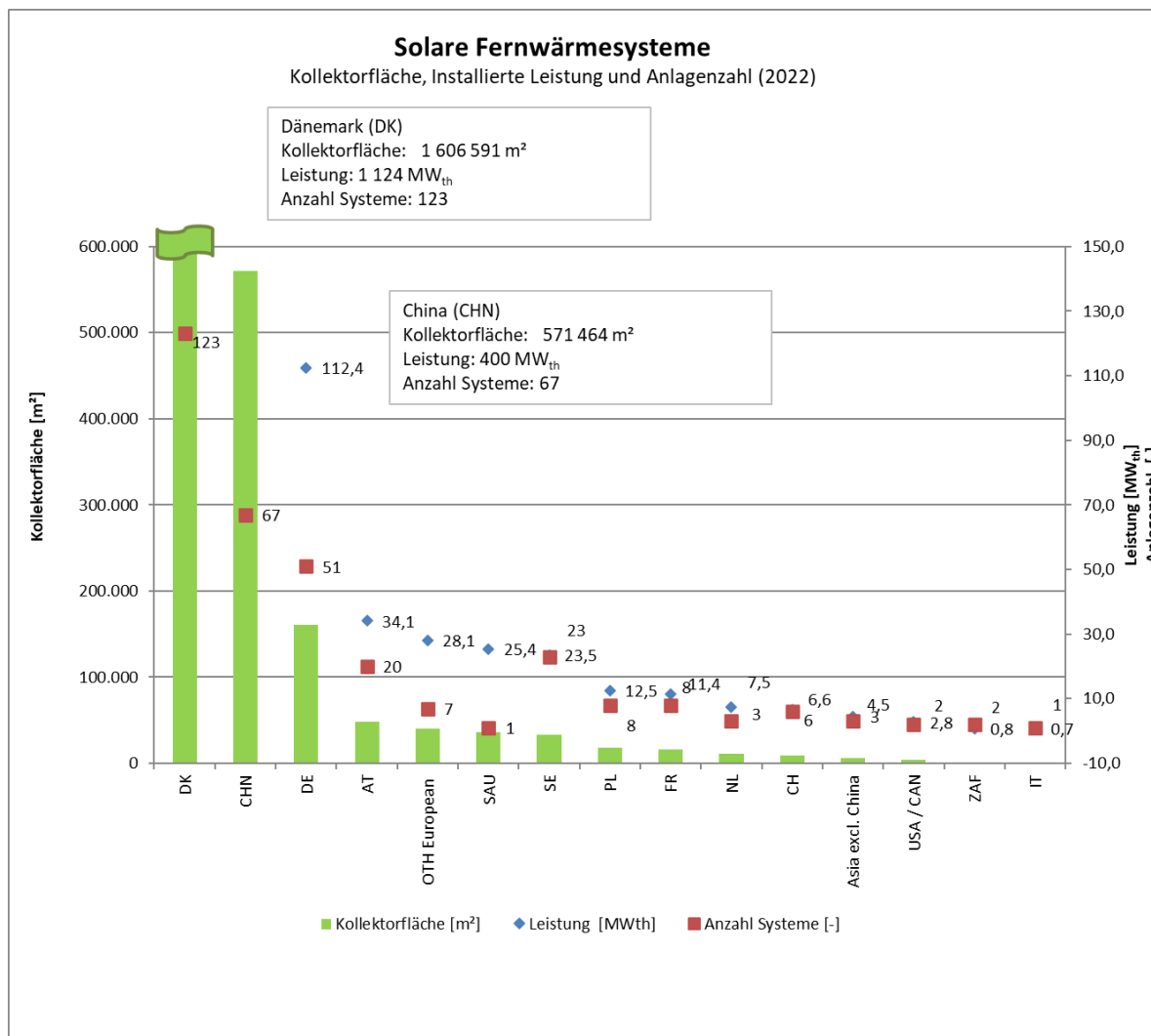
Abbildung 85 – Solare Fernwärmesysteme Leistungen und Kollektorfläche installiert sowie Anzahl der Anlagen im Jahr 2022 (alle Anlagen größer 500 m 2 Kollektorfläche bzw. 0,35MW th ). Quelle: Weiss, W., Spörk-Dür, M. (2023)
