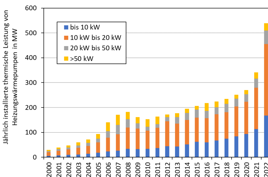
Abbildung 129 – Thermische Leistung neu installierter Heizungswärmepumpen in Österreich nach Leistungsklassen, für die Jahre 2000 bis 2022. Quelle: ENFOS (2023)
