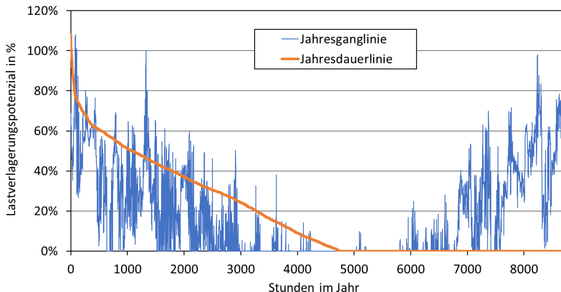
Abbildung 131 – Lastverlagerungspotenzial Gang- und Dauerlinie über ein Jahr auf Basis Testreferenzjahr Wr. Neustadt. Quelle: ENFOS (2023)
