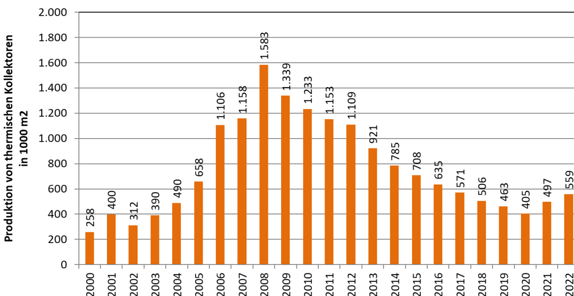
Abbildung 89 – Produktion von verglasten Flachkollektoren in Österreich
