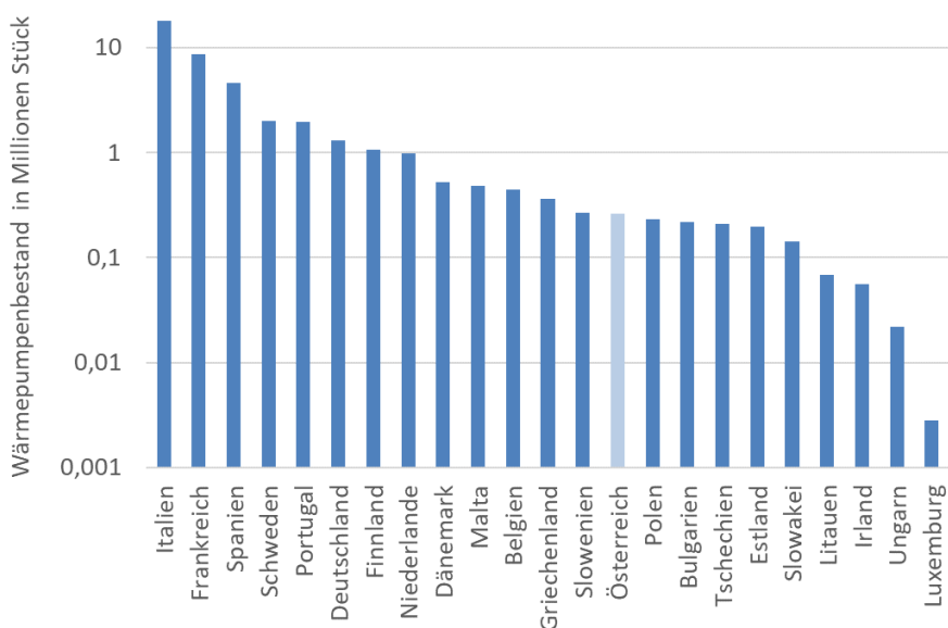
Abbildung 121 – Wärmepumpenbestand in den EU 27 Ländern im Jahr 2020
