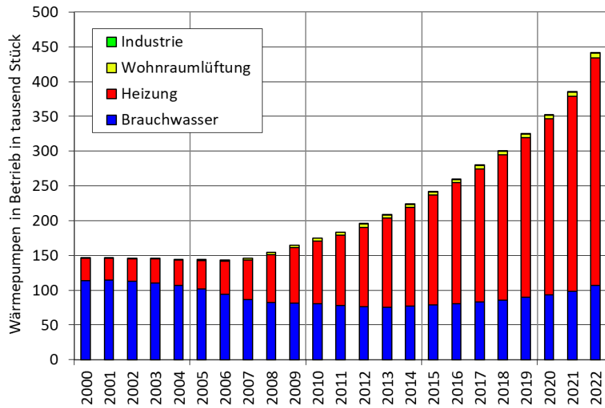
Abbildung 115 – Wärmepumpen-Bestandsentwicklung in Österreich bis 2022 Lebensdauer: 20 Jahre. Quellen: bis 2006: Faninger (2007), ab 2007: Biermayr et al. (2022), ENFOS (2023)
