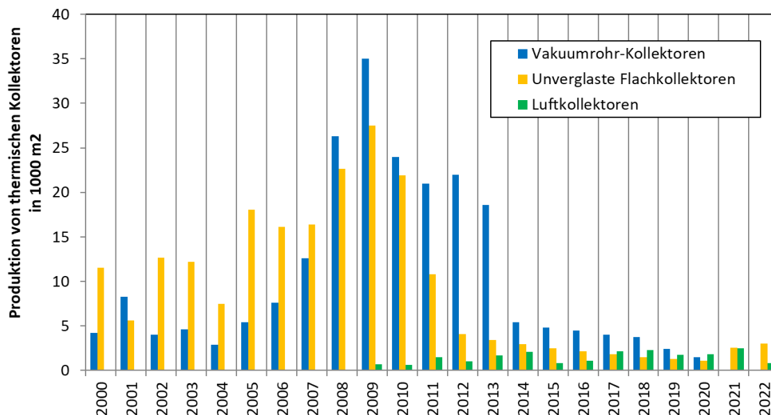
Abbildung 90 – Produktion von thermischen Solarkollektoren in Österreich Unverglaste Kollektoren, Vakuumrohr- und Luftkollektoren, in den Jahren 2000 bis 2022. Quellen: bis 2006: Faninger (2007), ab 2007: AEE INTEC (2023)
