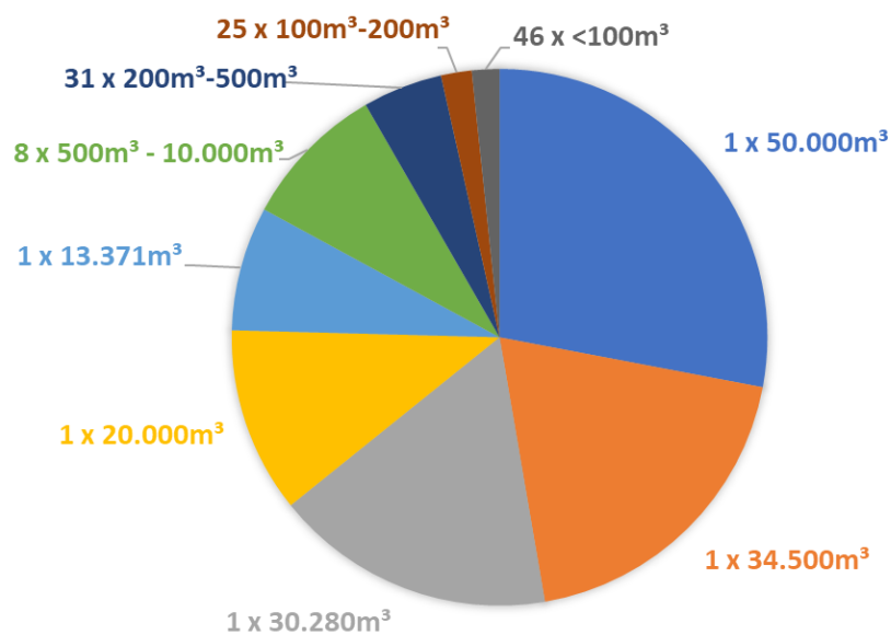
Abbildung 110 – Verteilung des Behälterspeichervolumens je Wärmenetz in den 200 größten Wärmenetzen (Datenbasis: 115 Wärmespeicher in 200 Wärmenetzen) Quelle: AEE INTEC (2023)
