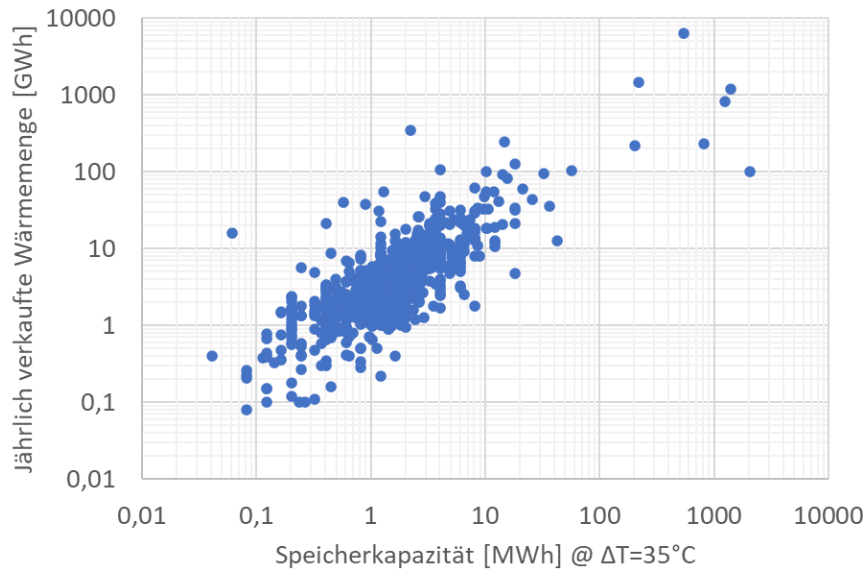
Abbildung 107 – Die jährlich verkaufte Wärmemenge je erhobenem Wärmenetz über der jeweils gesamt installierten Wärmespeicherkapazität Datenbasis: 702 Wärmenetze, Quelle: AEE INTEC (2023)
