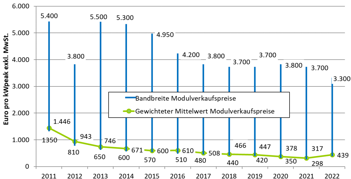
Abbildung 60 – Modulverkaufspreise österreichischer Modulhersteller 2011 bis 2022 Gewichteter Mittelwert und Bandbreite, Werte exkl. MWSt.; Anzahl der Nennungen: 2011: n=6, 2012: n=5, 2013: n=7, 2014: n=5, 2015: n=4, 2016: n=5, 2017: n=3, 2018: n=4 und 2019: n=3, 2020: n=3, 2021: n=3, 2022: n=3. Quelle: Technikum Wien (2023)
