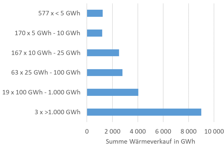
Abbildung 101 – Kategorisierung der erhobenen Wärmenetze auf Basis der verkauften Jahreswärmemenge (Datenbasis: 999 Wärmenetze) Quelle: AEE INTEC (2023)
