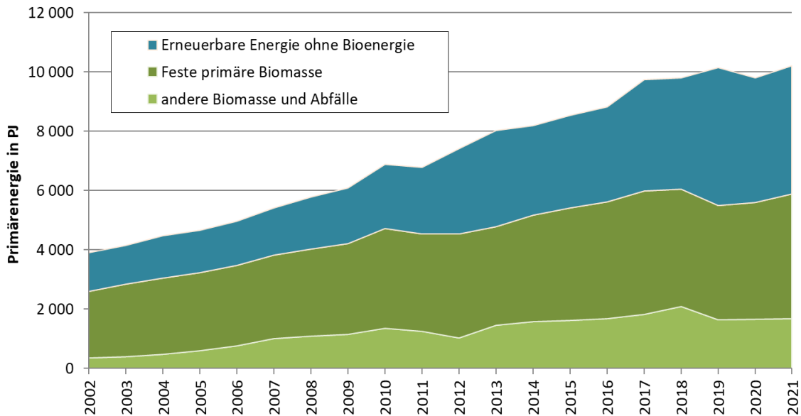
Abbildung 34 – Primärenergieerzeugung erneuerbarer Energie in den EU27 Staaten (bis 2019 EU28) in PJ. Quelle: Eurostat (2023a)
