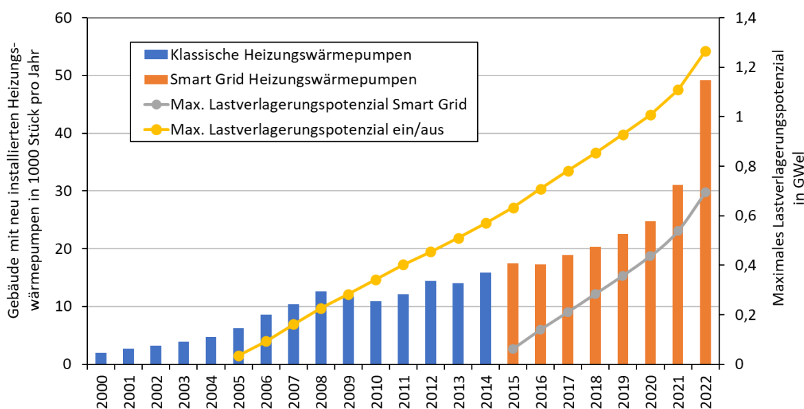
Abbildung 8 – Entwicklung des netzdienlichen Lastverlagerungspotenzials durch thermisch aktivierte Bauteile und Gebäude. Quelle: ENFOS (2023)
