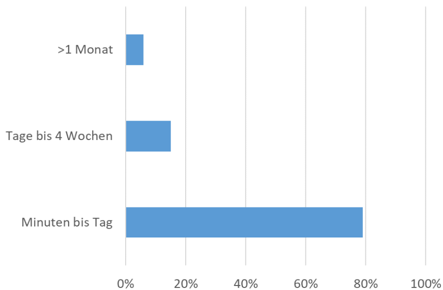
Abbildung 109 – Zuteilung der Wärmespeicher nach Speicherdauer Datenbasis: 104 Angaben für 88 Wärmenetze, Mehrfachnennungen je Netz möglich Quelle: AEE INTEC (2023)
