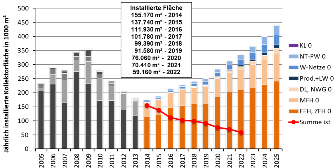
Abbildung 95 – Jährliche Kollektorfläche: „Forcierte Aktivitäten“ Szenario und Realität Quelle: Fink et al. (2014)
