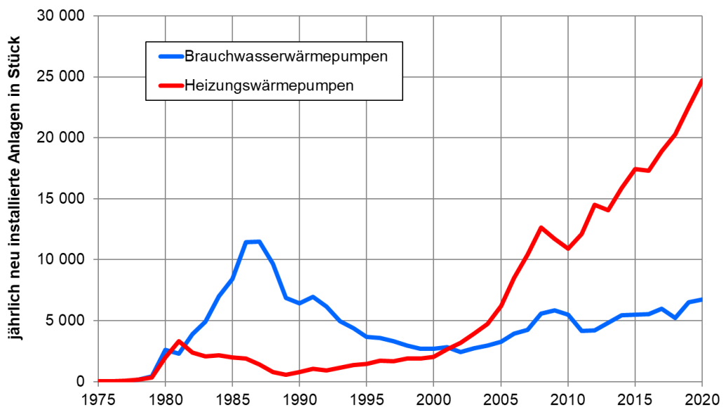
Abbildung 85 – Brauchwasser- und Heizungswärmepumpen in Österreich bis 2020 Quellen: bis 2006: Faninger (2007), ab 2007: Biermayr et al. (2008 ff), ENFOS (2021)
