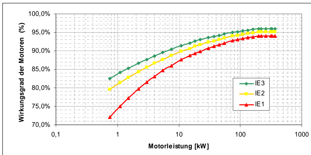
Abbildung 2 Wirkungsgradanforderungen für Elektromotoren (als Beispiel für 4-polige AC-Motoren) lt. IEC Standard 60034-30, eigene Darstellung
