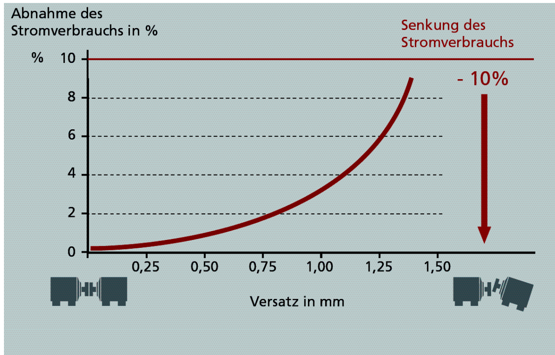
Abbildung 7 Zusammenhang Stromverbrauchsanstieg in Prozent mit dem Versatz in mm (Quelle: www.pruftechnik.com )
