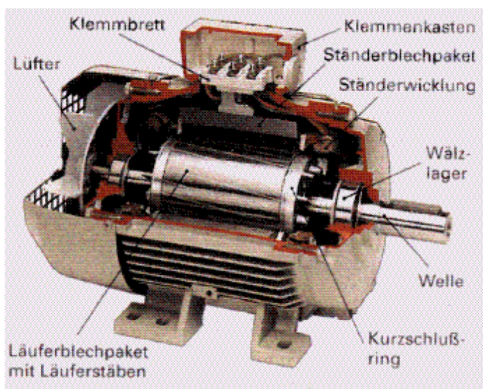
Abbildung 4 Komponenten eines Drehstrom-Asynchronmotors, (SEW Eurodrive, 2004, S4)
