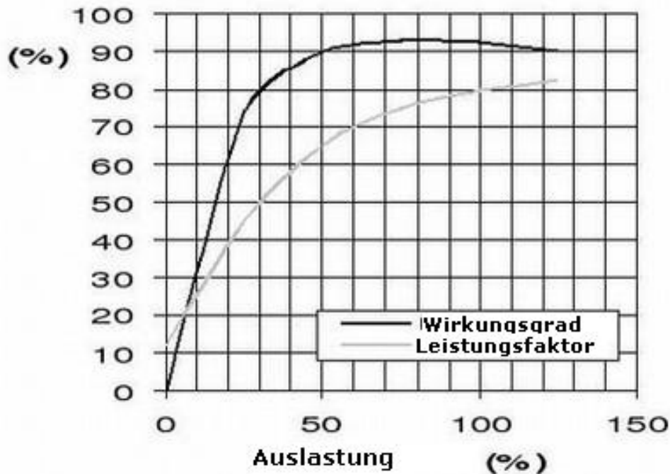
Abbildung 6 Zusammenhang Wirkungsgrad, Leistungsfaktor und Auslastung eines AC-Motors
