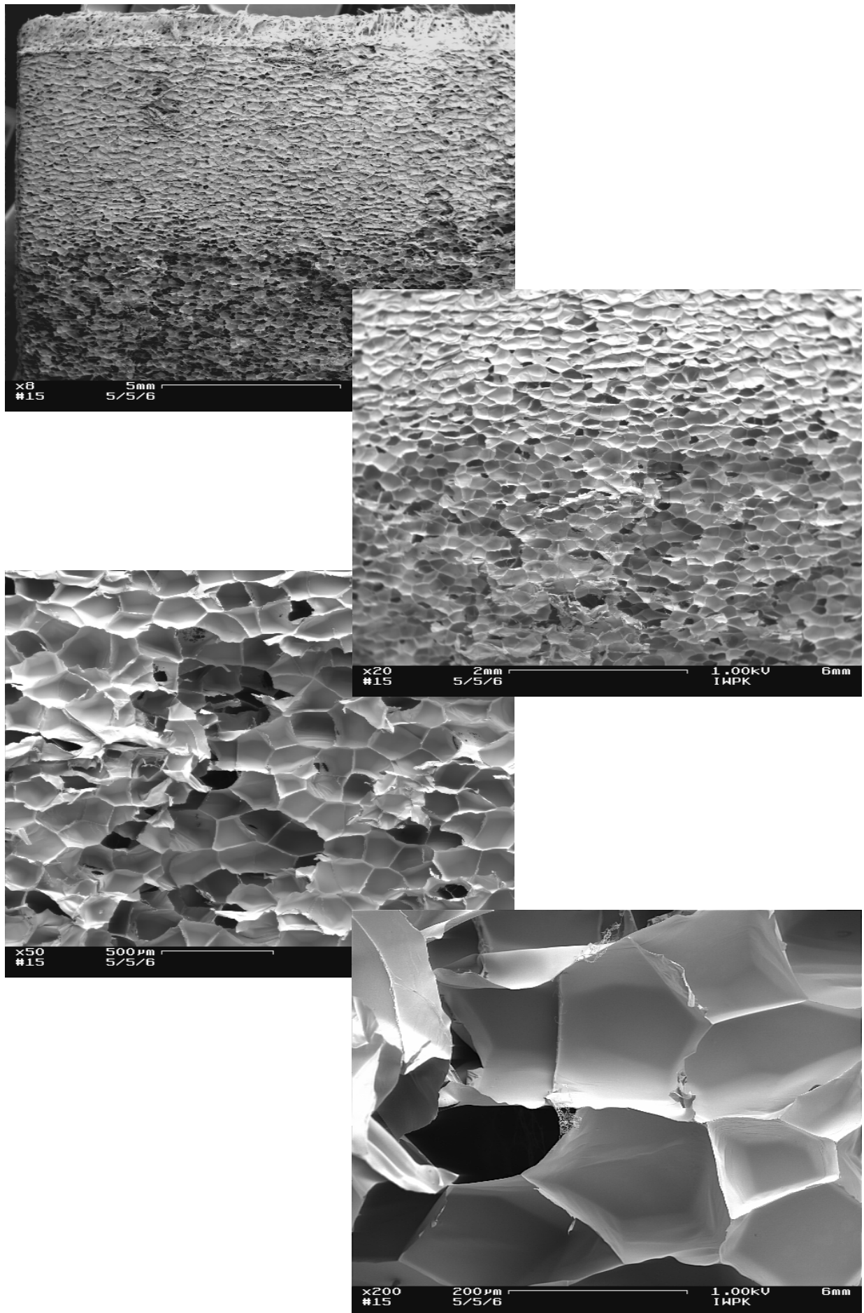
Abb. 3-33: Überblick über den mittels REM untersuchten Probekörper für XPS-R035.
