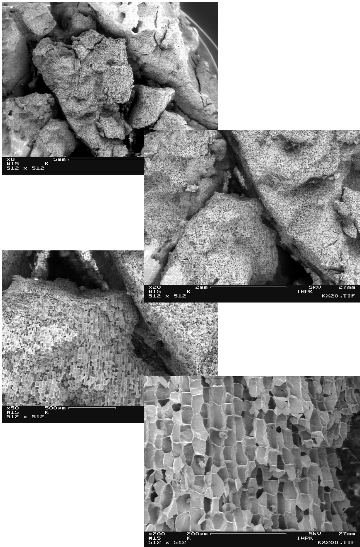
Abb. 3-34: Überblick über den mittels REM untersuchten Probekörper für Kork.
