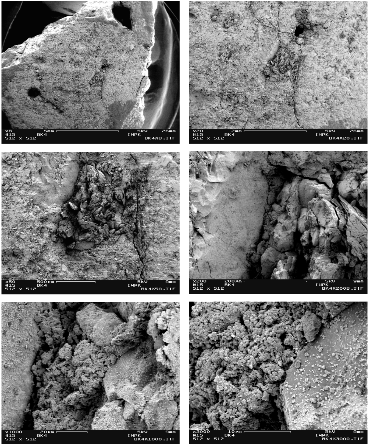
Abb. 3-36: Überblick über den mittels REM untersuchten Probekörper für Beton K4.
