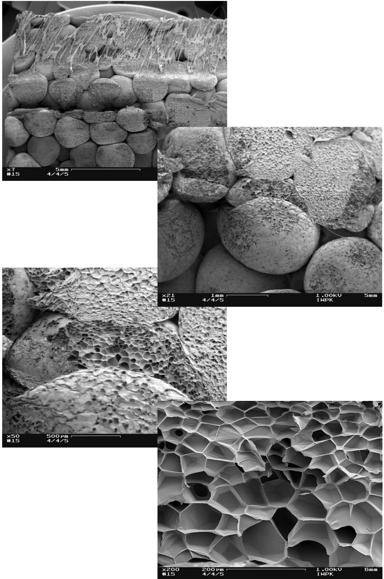
Abb. 3-32: Überblick über den mittels REM untersuchten Probekörper für EPS-W30.
